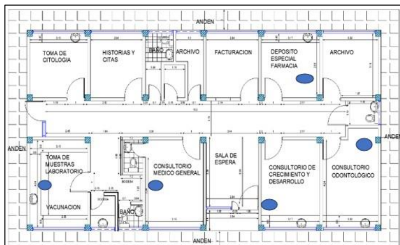
Ilustración 15. Ubicación de puntos a 220V.
