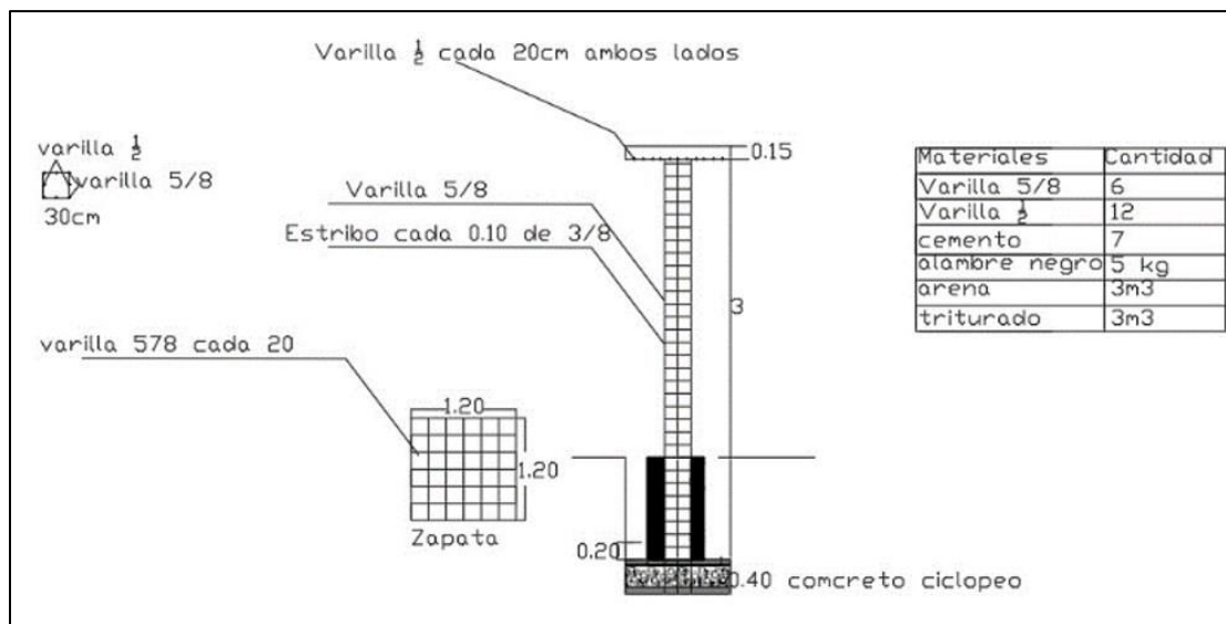
Ilustración 21. Diseño de la columna con su respectiva placa
