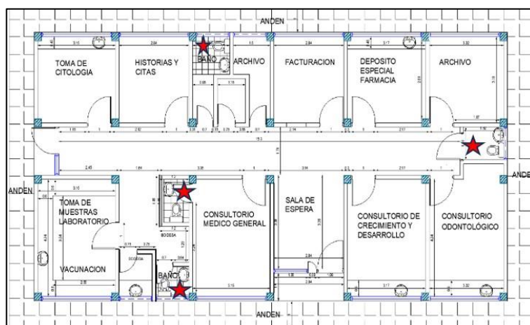
Ilustración 18. Ubicación de los accesorios de baño
