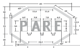
Figura 2-7. Dimensiones sugeridas para postes de señales verticales
