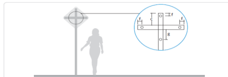
Figura 2-7. Dimensiones sugeridas para postes de señales verticales
