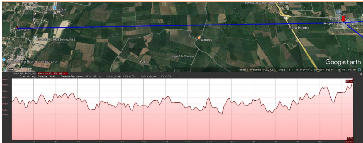
Ilustración 1 Perfil radio enlace Calipuerto-Aeropuerto Alfonso Bonilla Aragón
