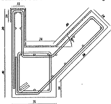
DETALLE VIGA CANAL
