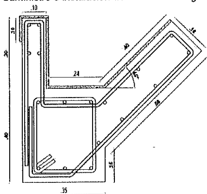
DETALLE VIGA CANAL ESCALA 1:10
