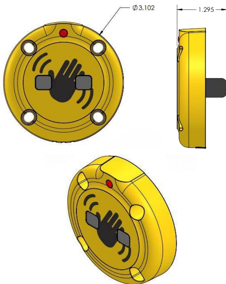
Se muestra el modelo 4EVR® MOAB Wave
