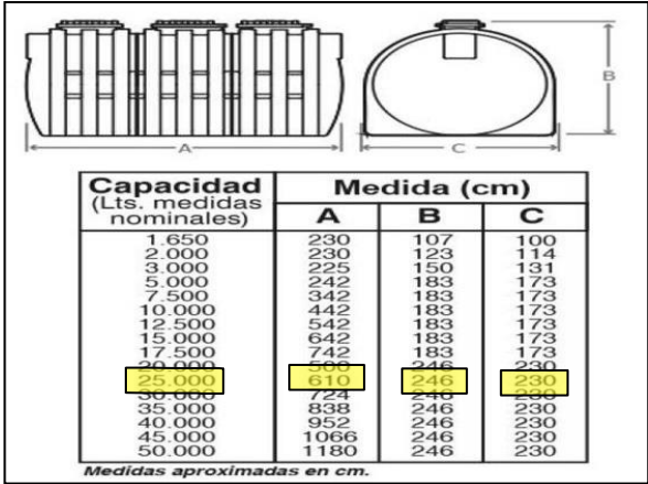
Imagen 4: Tanque séptico. Volumen y dimensiones.
