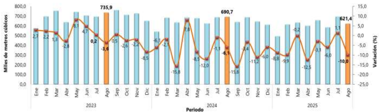
Gráfico 2. Producción de concreto premezclado (miles de metros cúbicos y variación anual) Total nacional Enero 2023 – agosto 2025 P
