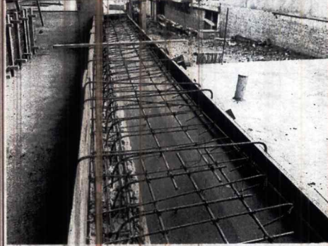
FOTO 11: Armado de acero para alfajias
