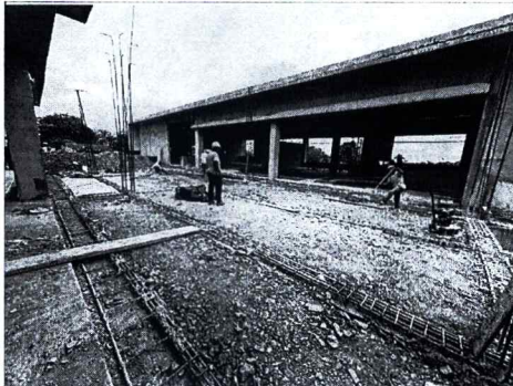
FOTO 2: relleno de material de subase para losa pasarela entepiso 3
