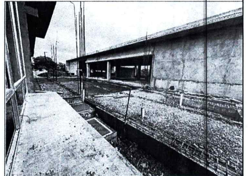
FOTO 3: Plastico negro para islar material de acuerdo al diseño pasarela 3
