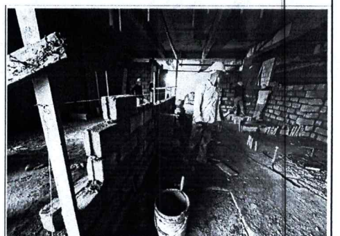
FOTO 9: Levante bloque n 12, relleno para los muros de subestacion
