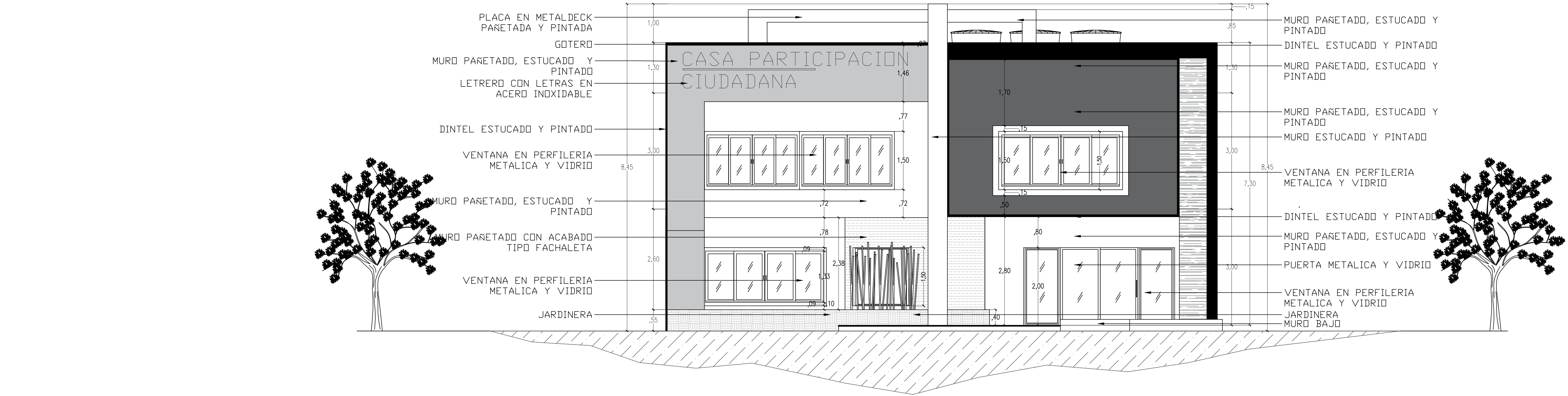
FACHADA FRONTAL ESC_1:50
