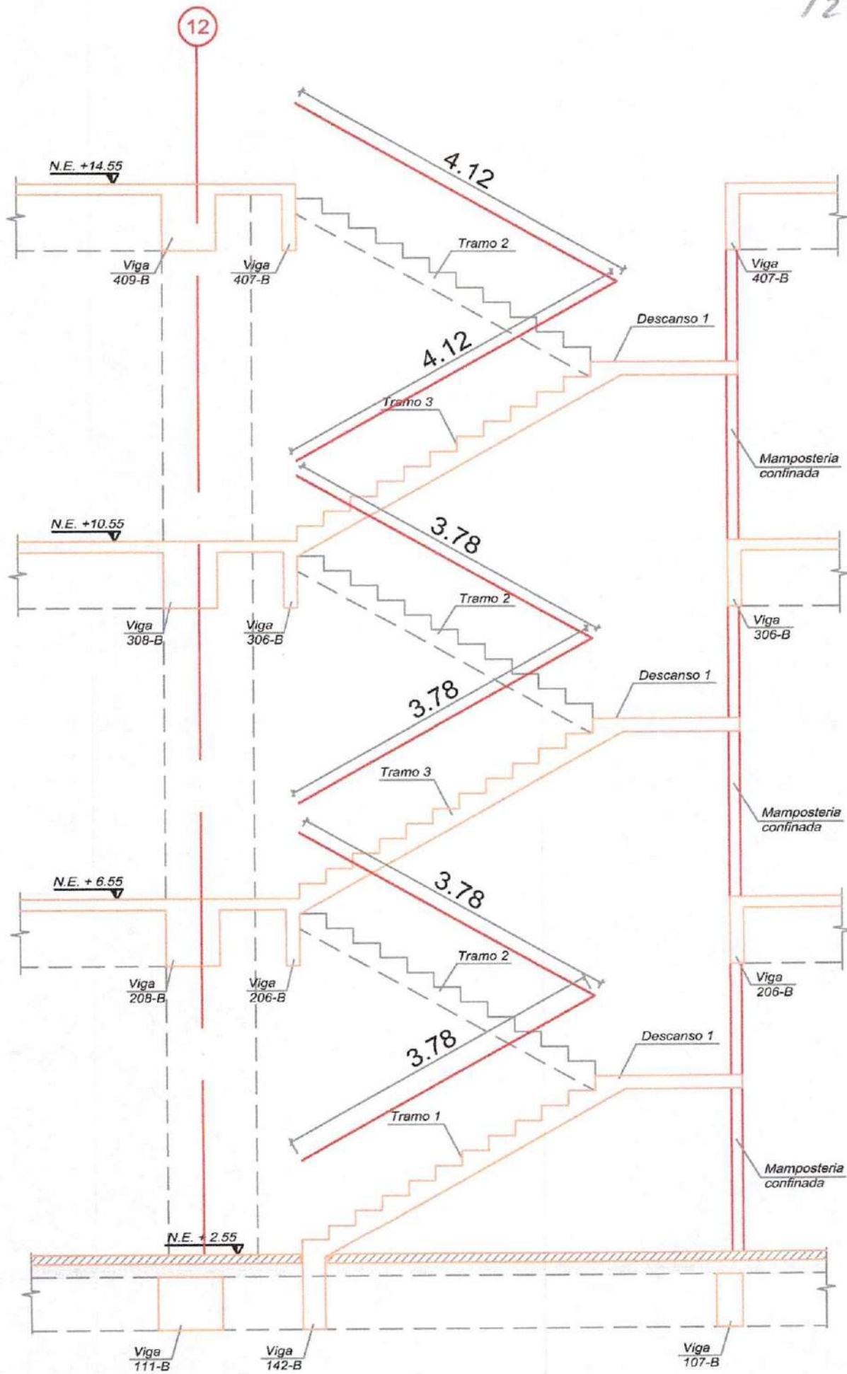
ALZADO GENERAL DE ESCALERA E-3 Escala 1:50
