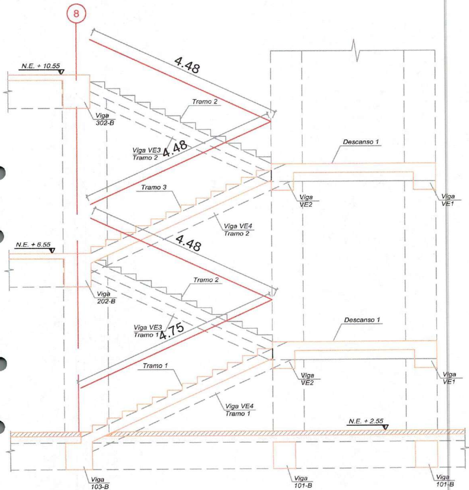
ALZADO GENERAL DE ESCALERA E-1 Escala 1:50
