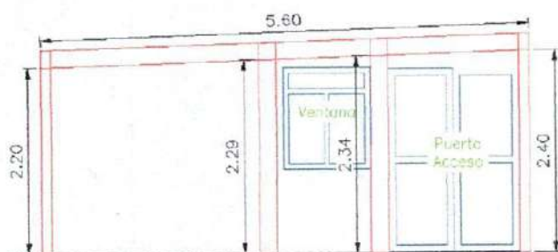
FACHADA 1
