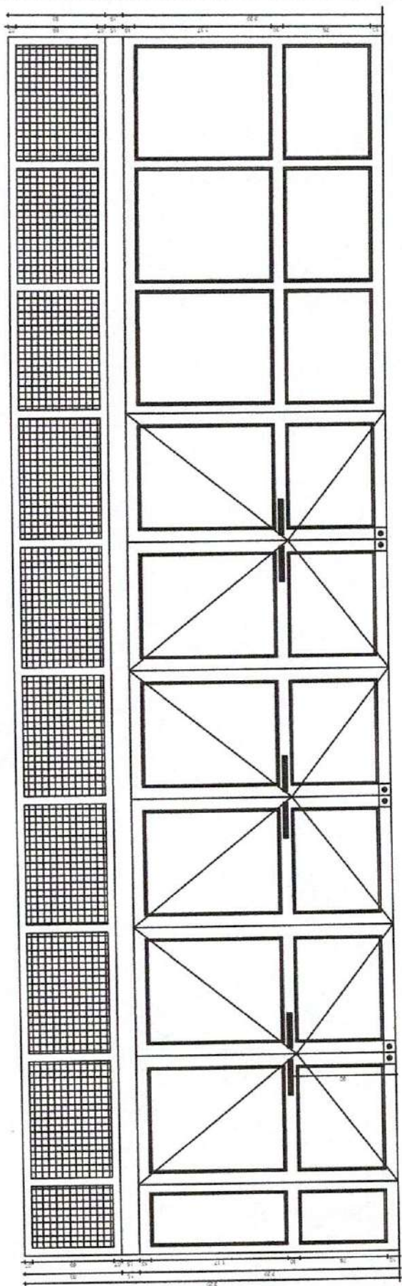
ALZADO EXTERIOR
