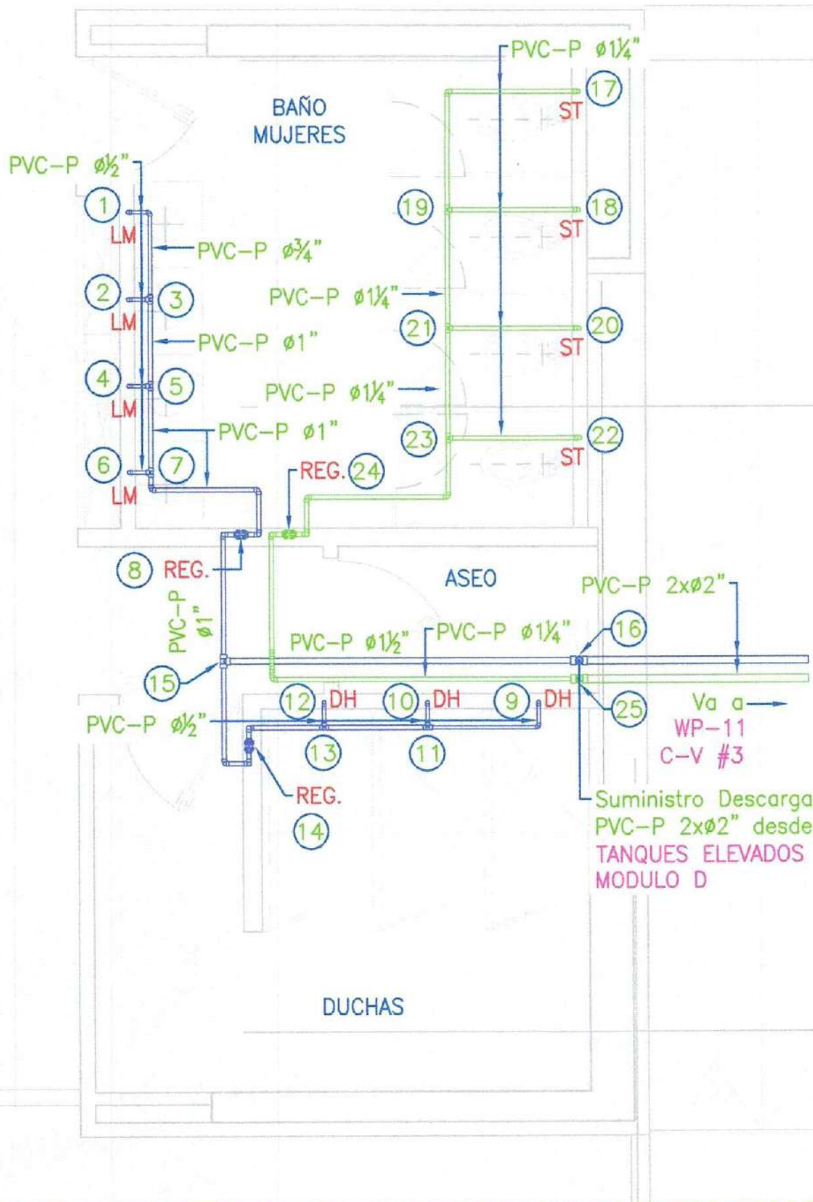
DETALLE - F1 PLANTA GENERAL Escala 1:50
