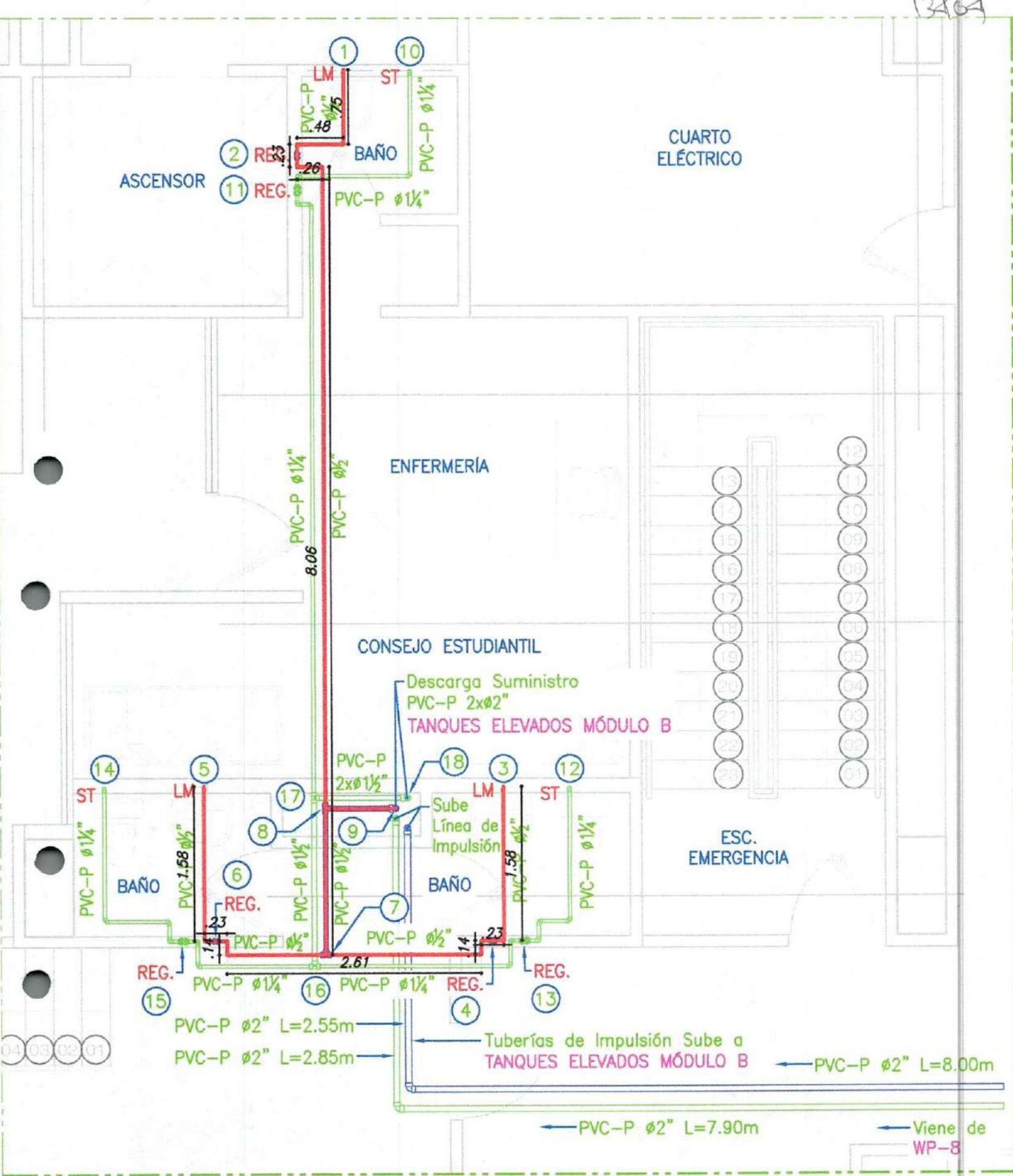
DETALLE - C1 PLANTA GENERAL Escala 1:50
