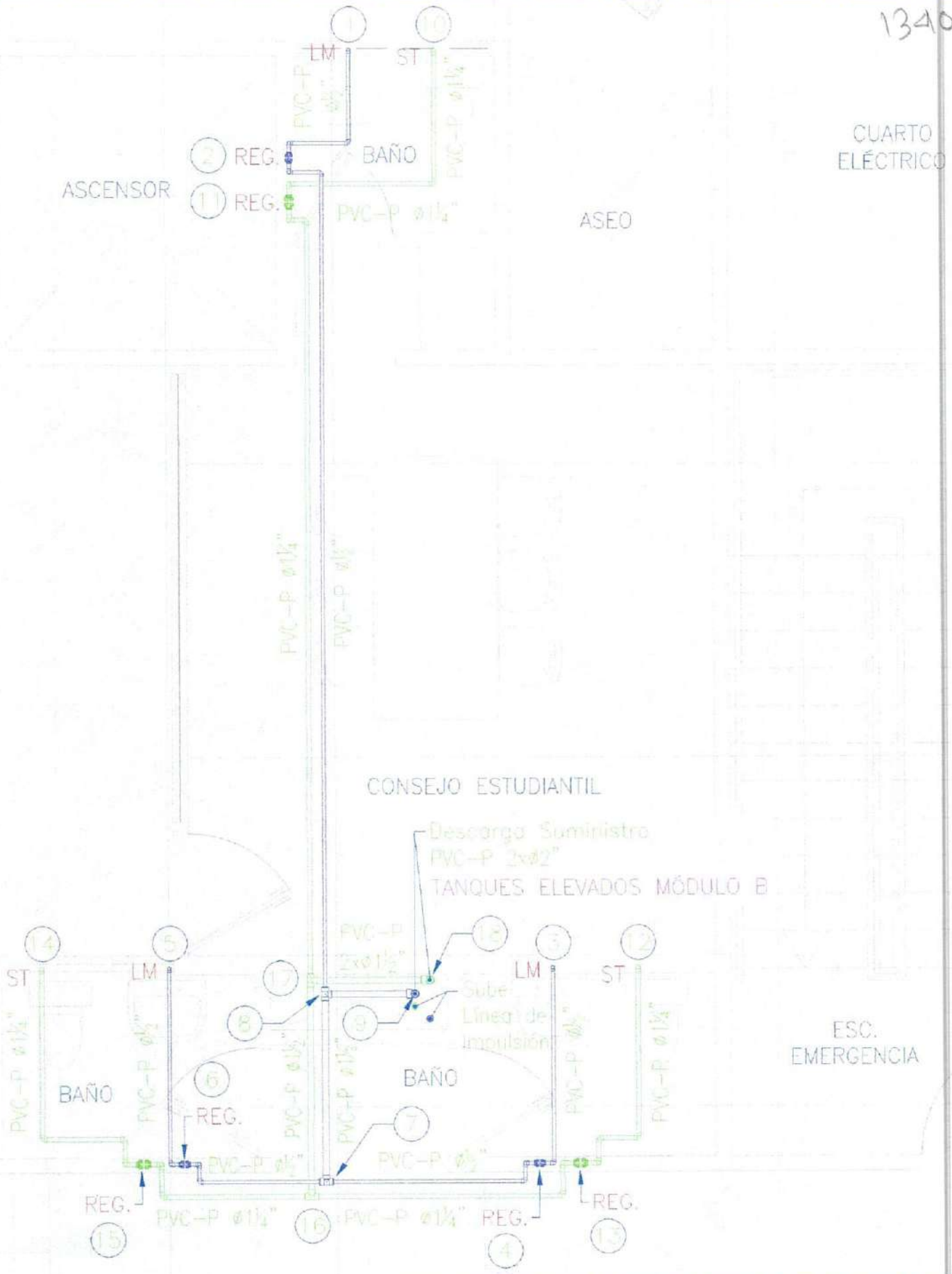
PLANTA GENERAL Escala 1:50
