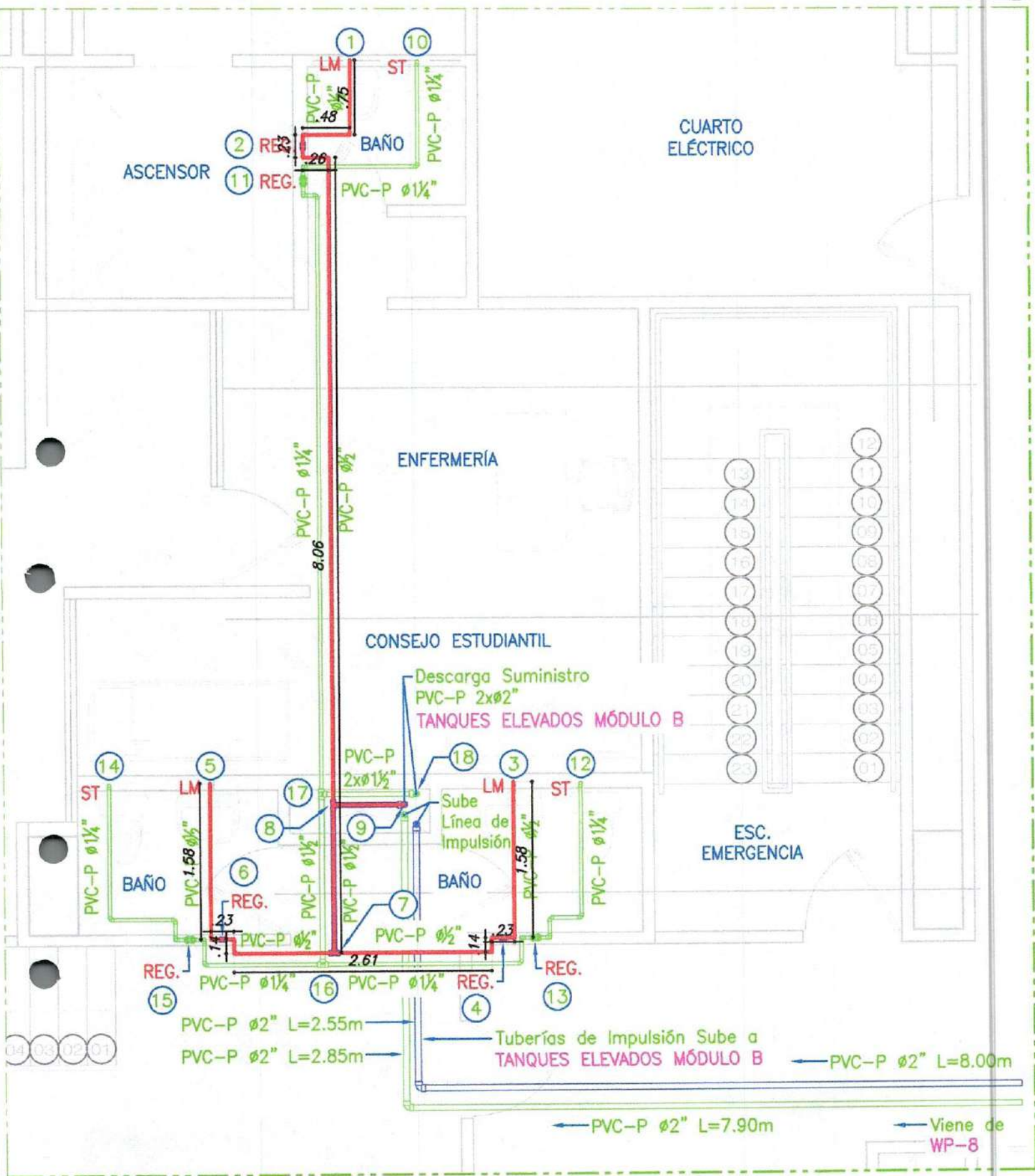
DETALLE - C1 PLANTA GENERAL Escala 1:50
