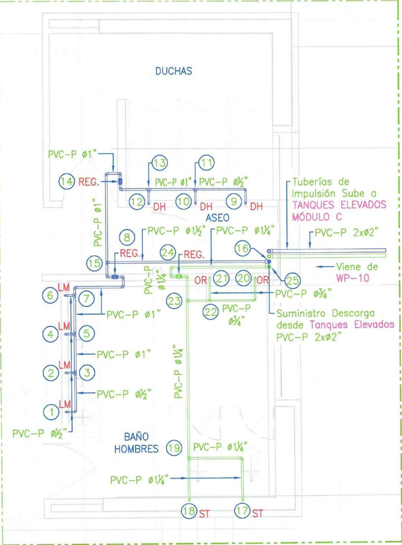
DETALLE - E1 PLANTA GENERAL Escala 1:50
