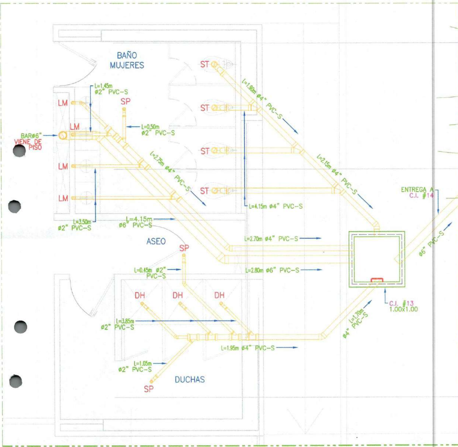
DETALLE - F1 Escala 1:50
