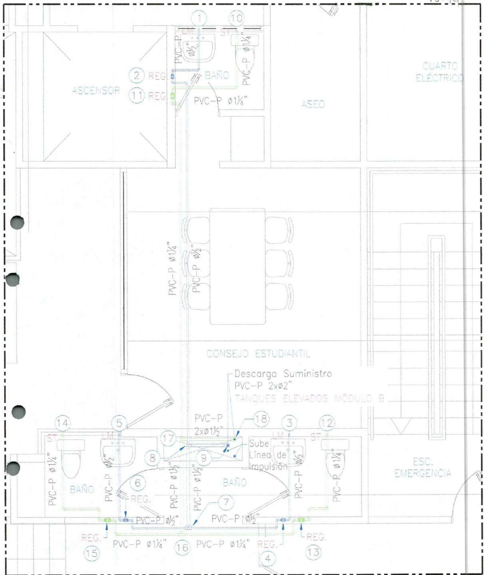
DETALLE — B2 PLANTA GENERAL Escala 1:50
