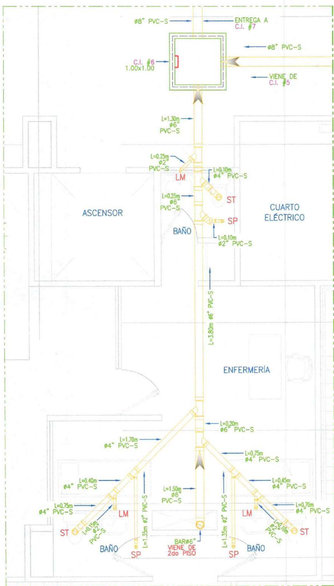
DETALLE - D1 Escala 1:50
