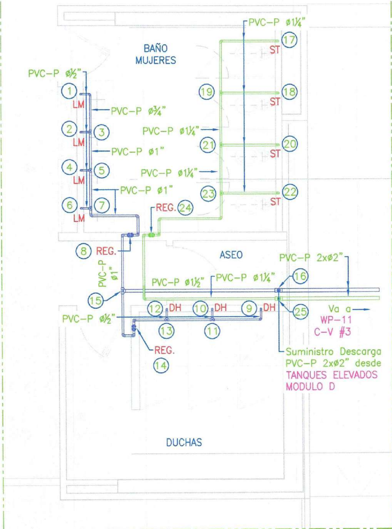
DETALLE - F1 PLANTA GENERAL Escala 1:50
