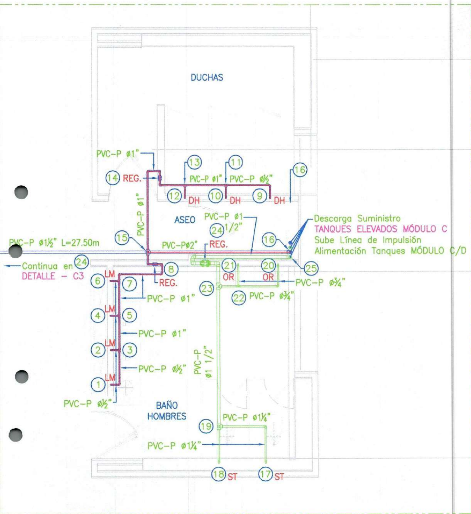
DETALLE - D3 PLANTA GENERAL Escala 1:50
