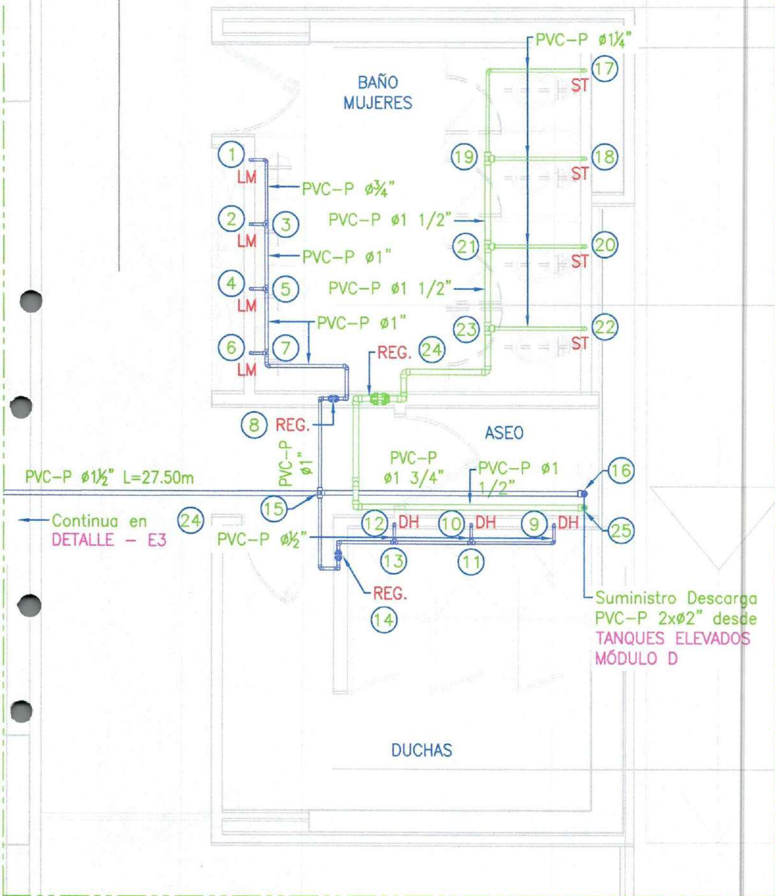
DETALLE - F3 PLANTA GENERAL Escala 1:50
