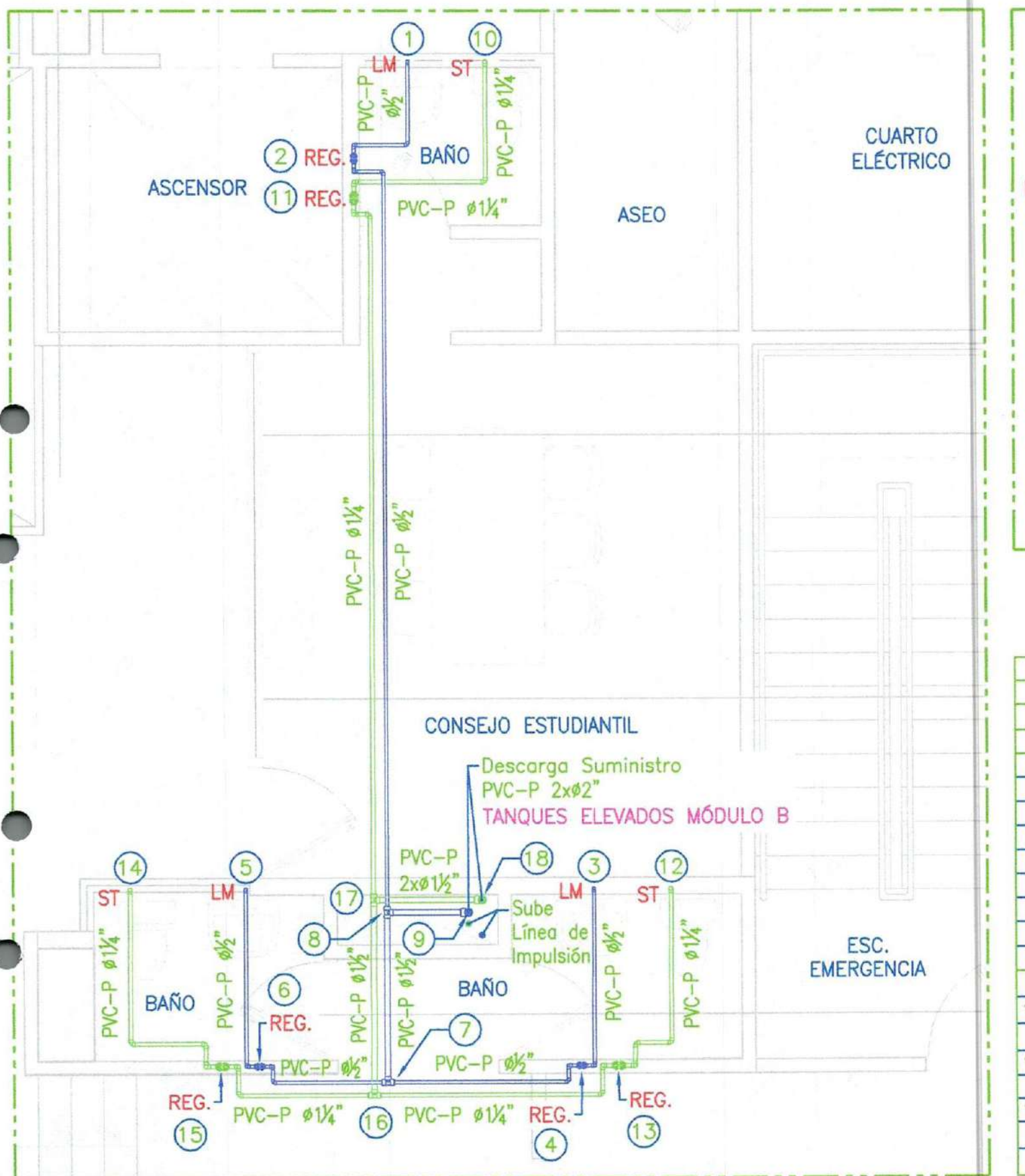
DETALLE - B2 PLANTA GENERAL
