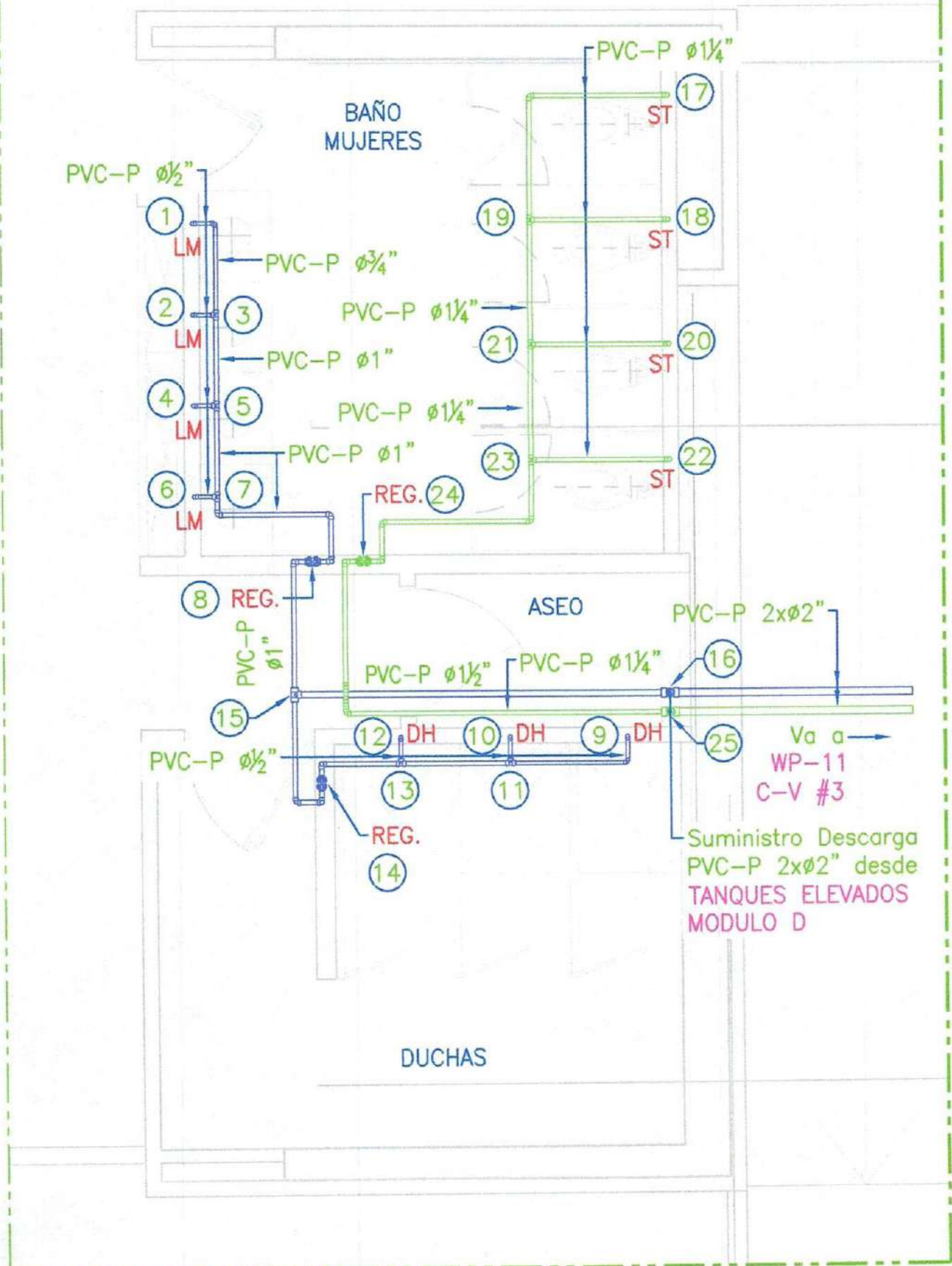
DETALLE - F1 PLANTA GENERAL Escala 1:50
