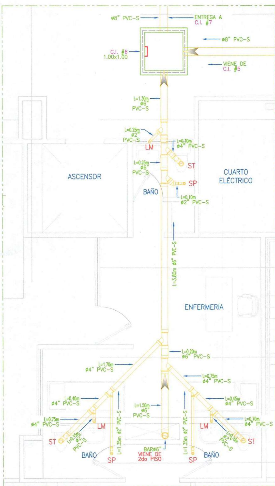
DETALLE - D1
