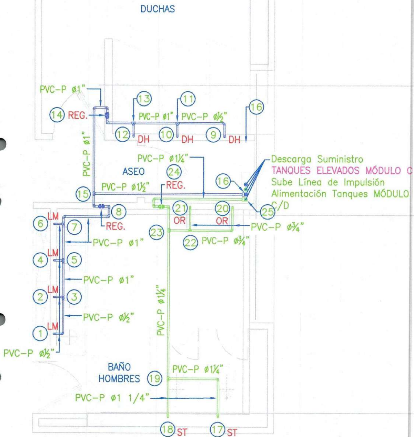
DETALLE - D2 PLANTA GENERAL Escala 1:50
