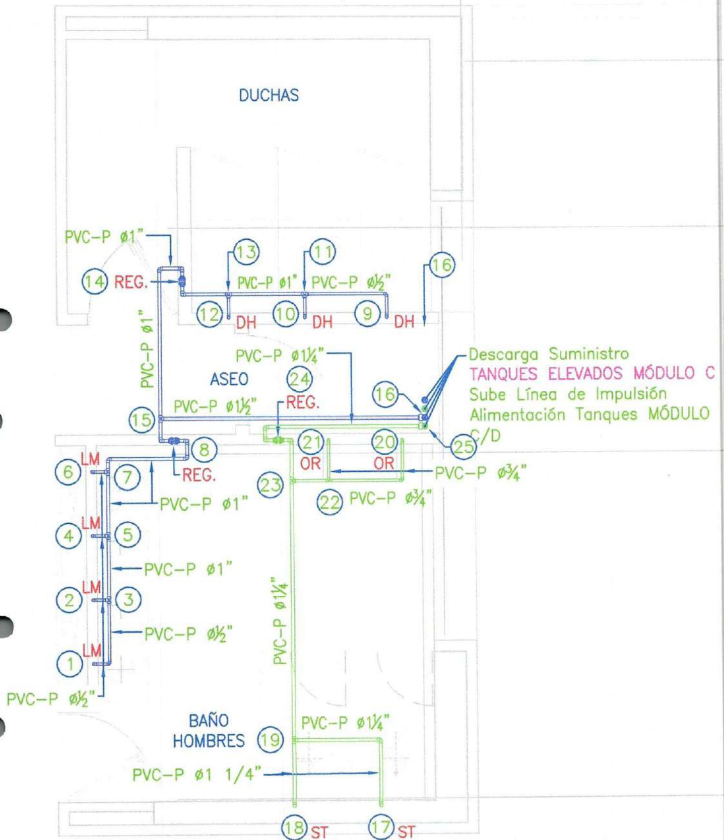
DETALLE - D2 PLANTA GENERAL Escala 1:50
