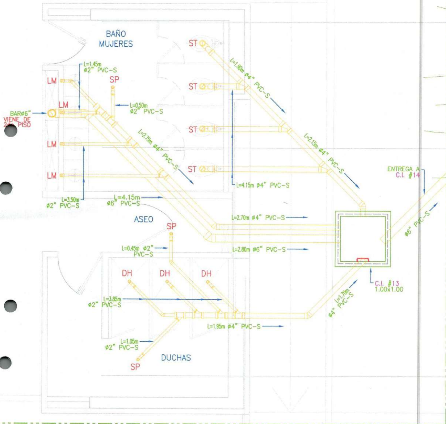
DETALLE - F1
