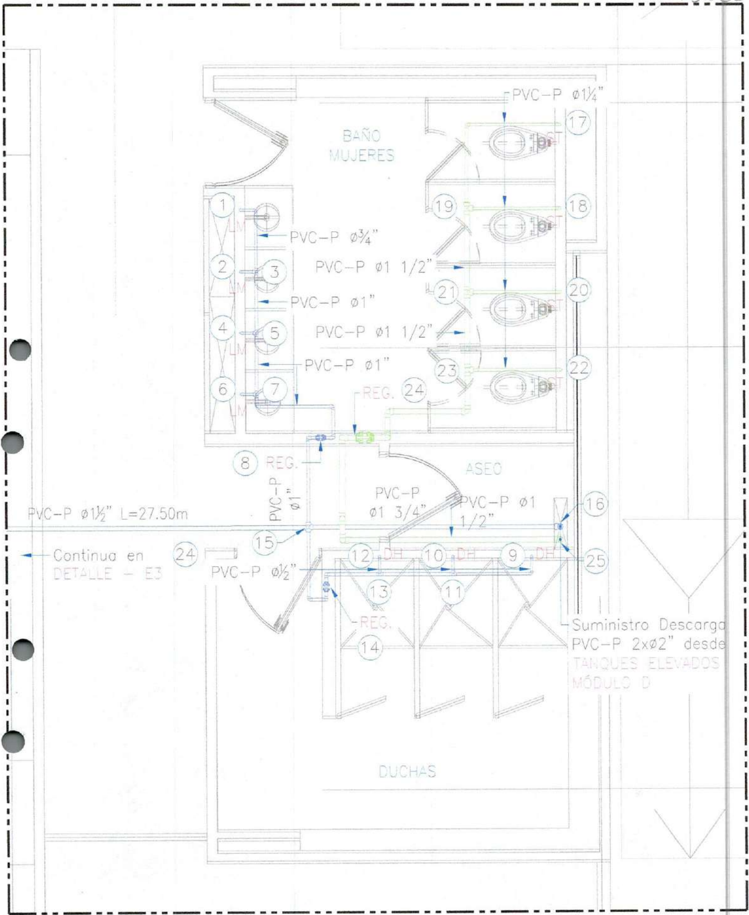
DETALLE - F3 PLANTA GENERAL Escala 1:50
