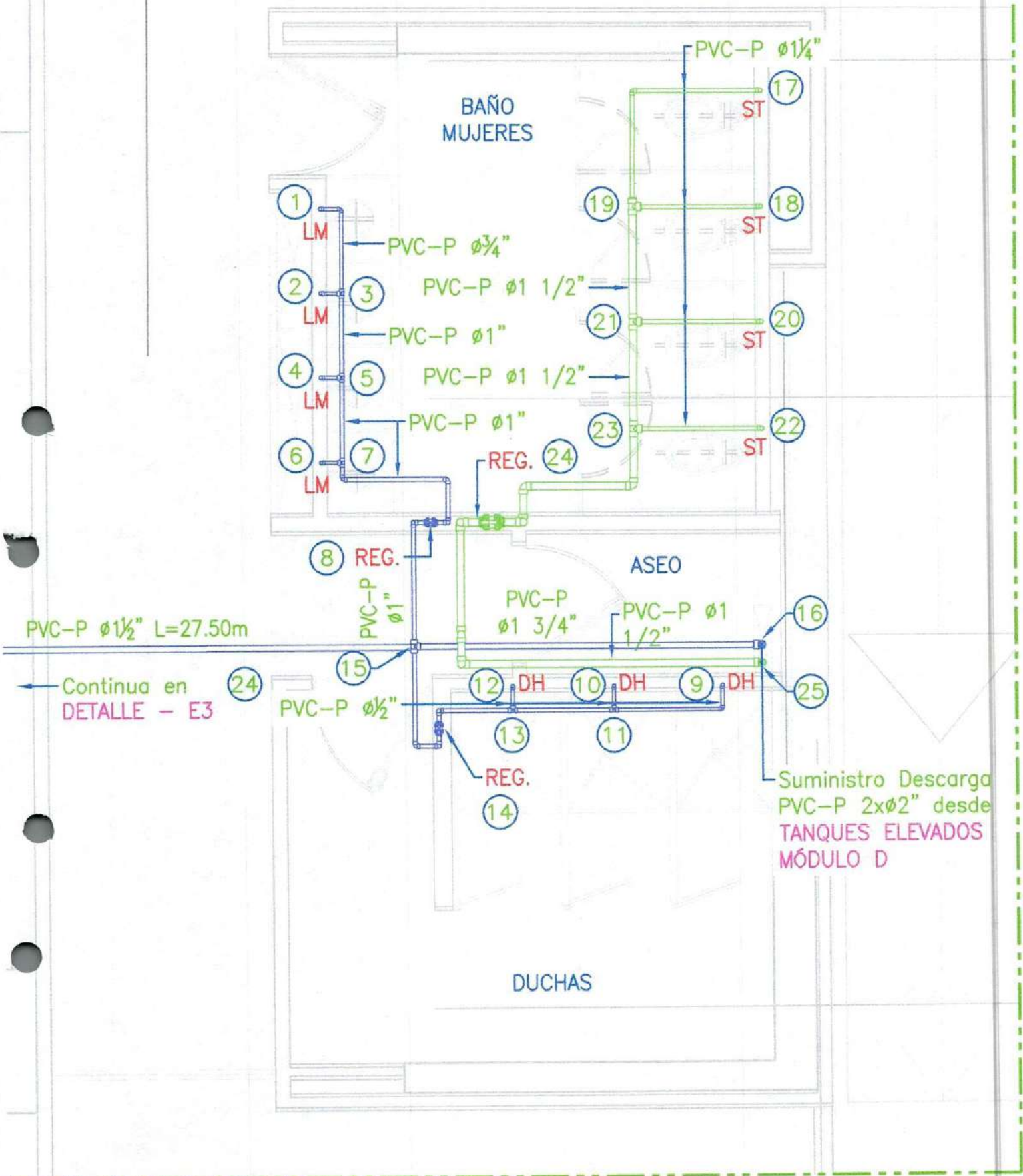
DETALLE - F3 PLANTA GENERAL Escala 1:50
