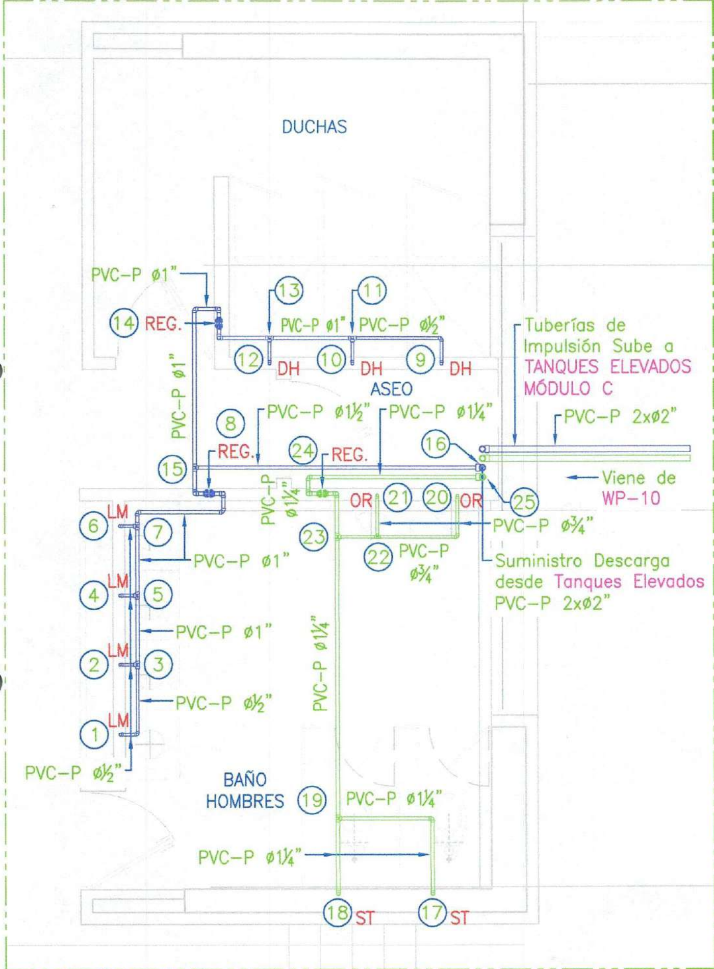
DETALLE - E1 PLANTA GENERAL Escala 1:50
