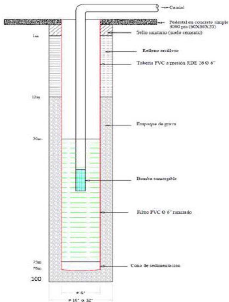
Figura 8.1 Pozo SENA, Angostura, diseño preliminar
