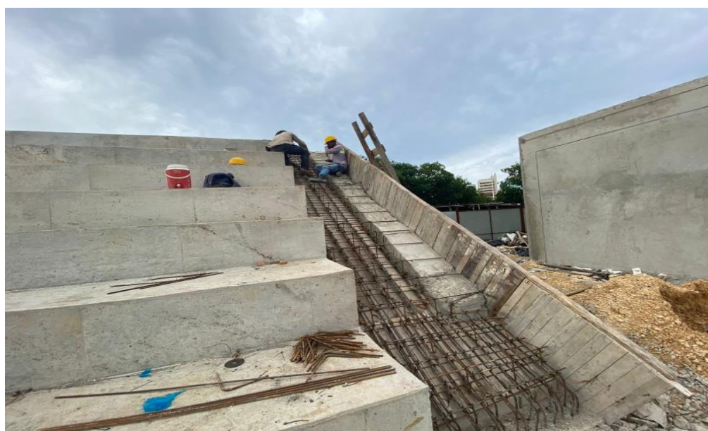
Ilustración 16. Figurado acero 60000 psi para escaleras graderías de softbol
