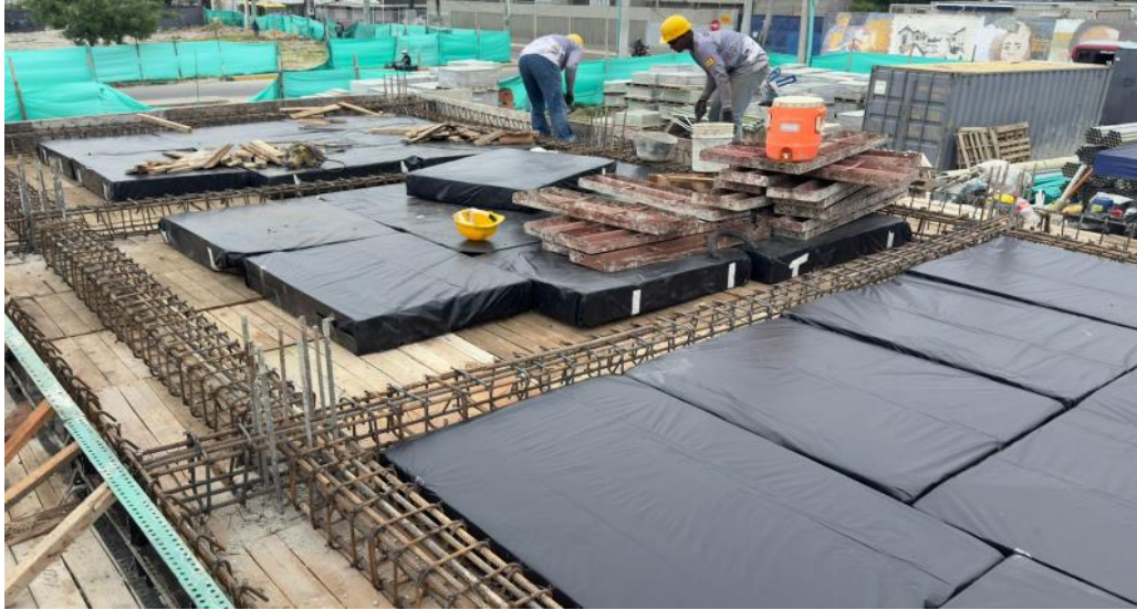
Ilustración 37. Figurado acero de refuerzo 60.000 placa cuartos técnicos
