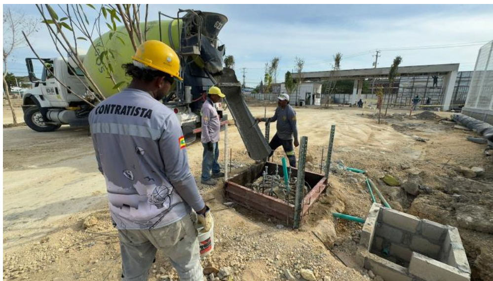
Ilustración 44. Fundida concreto 4000 psi para mástiles de iluminación canchas
