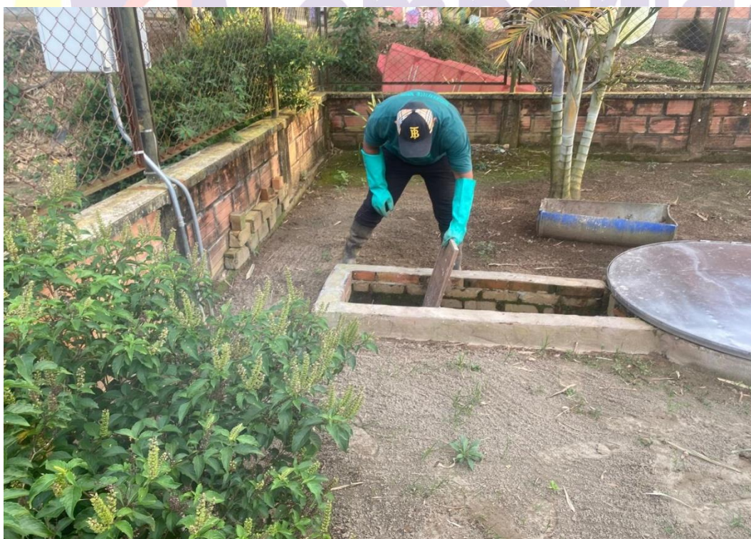
Limpieza y lavado de rejillas del sistema de cribado.
