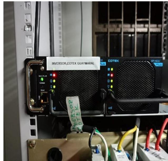
Foto 4. reubicación del sistema de inversor red ATN
