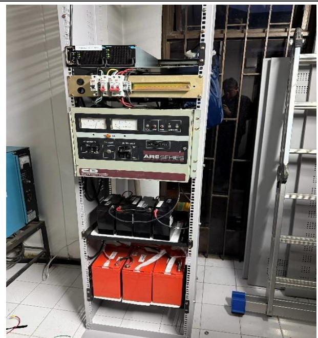
Foto 8. Equipos de energía reubicados en cuarto eléctrico del primer piso
