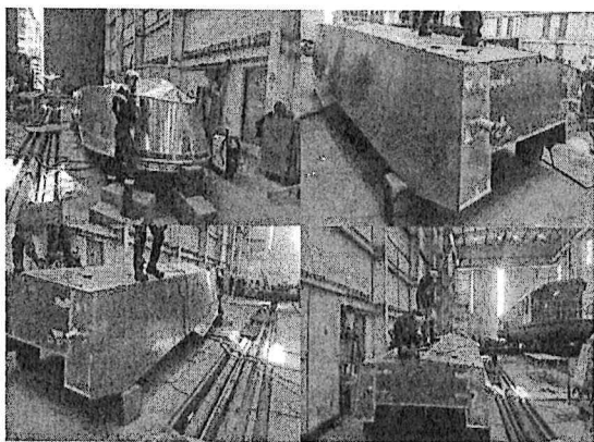
Foto No. 17 a 20 – Bote No. 25 Refuerzos cuadernas y vagras
