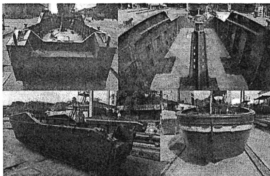
Foto No. 94 a 97 – Bote No. 23 y N° 24 Aplicación de esquema de pintura
