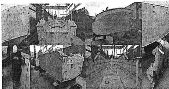
Foto No. 69 a 74 – Bote No. 23 y N°24 Finalización de proceso de granallado
