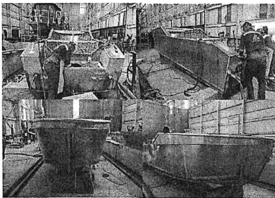
Foto No. 47 a 50 – Bote No. 26 Refuerzos, tuberías, forro del casco, espejo y verduguillo
