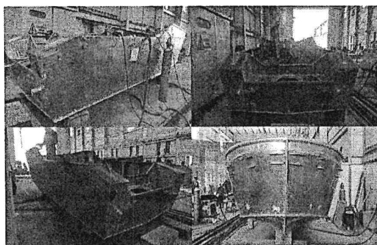
Foto No. 75 a 78 – Bote No. 25 Proceso de construcción
