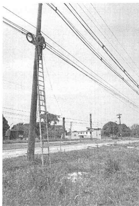
Ilustración 2 Instalación de fibra óptica en poste exterior 2
