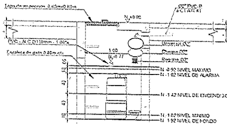
CORTE A-A POZO EYECTOR AGUAS RESIDUALES
