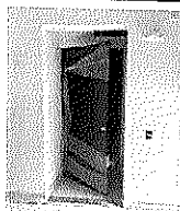
P-2 PUERTA BAOO PARA PERSONAS EN CONICION DE DISCAPACIDAD METALICA MARCO Y TABLERO LAMINA COLD ROLLED CAL 18 ANTICORROSIVO + ISMATEL CLERADURA DE SEGURIDAD LLAVE AL EXTERIOR, MANIPULOSA AL INTERIOR
