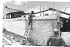
PANETE IMPERMEABILIZADO MUROS 1.3, 1.4-1.5 CM (LIBRAL)
