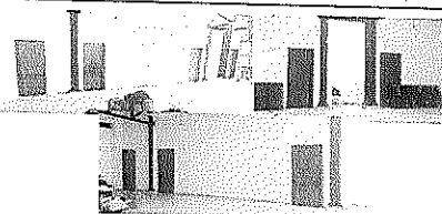
M-7 PUERTA BATIENTE, - EN MADERA ENTAMBUADA TUBO 1.8 X 0.7M, 1.0M, MARCO EN MADERA 0.20M CLERADURA ENTRADA PRINCIPAL Y BARRA ANTIBRAZO
