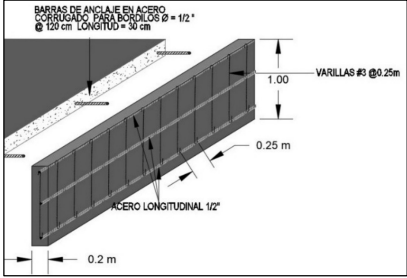
SECCION TIPICA BOX
