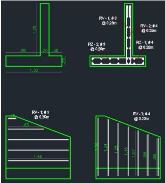
REFUERZO TIPICO ALETAS
