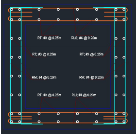
REFUERZO TIPICO BOXSENCILLO
