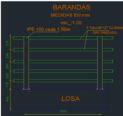
BARANDA METALICA
