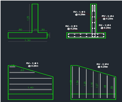
REFUERZO ALETAS BOX DOBLE
