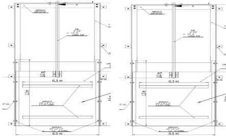
DISEÑO DE COMPUERTAS
