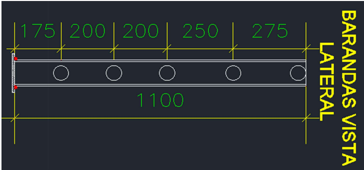
PLANTA BARANDA
