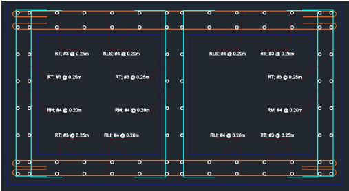
SECCION TIPICA REFUERZO BOX DOBLE
