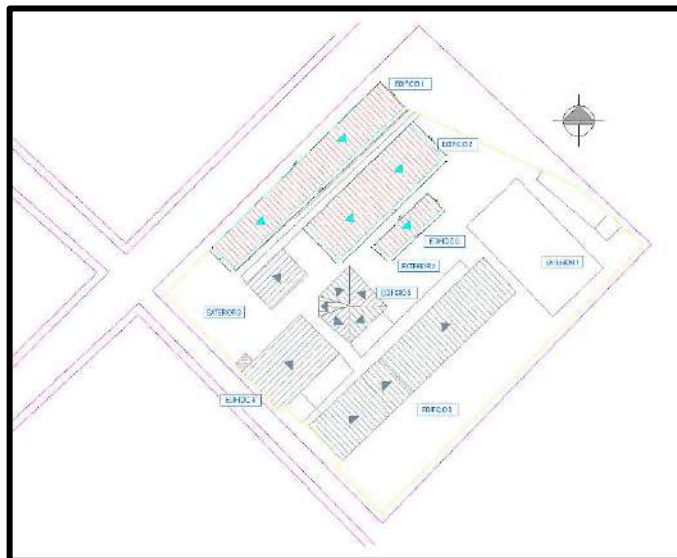
Ilustración 9. Esquema de Distribución Colegio Brasília Sede A Fuente: Propia
