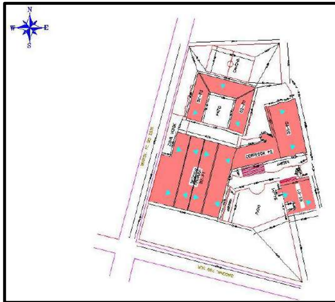
Ilustración 5. Esquema de Distribución Colegio Miguel de Cervantes Saavedra Sede A Fuente: Propia
