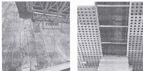
Fig. 6-7 Unión Losa - Rampa (raads) y vista interna superior de la junta Losa - Rampa
