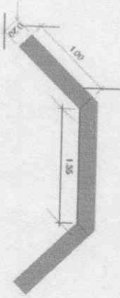
DETALLE DE CABEZALES PARA OBRAS DE ALCANTARILLADO
