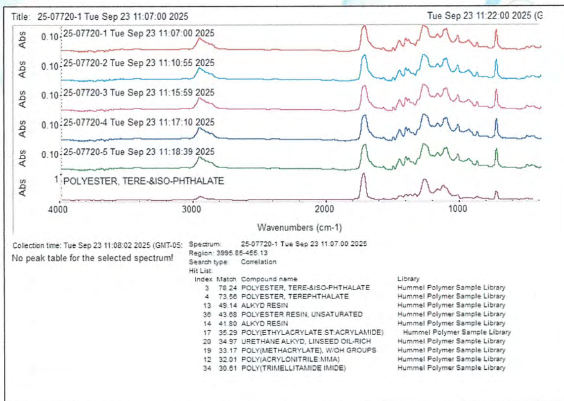
Grafica 1. Análisis FTIR
