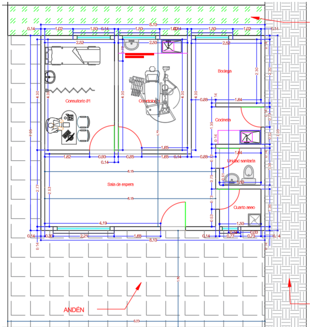
PLANTA ARQUITECTONICA PUESTO DE SALUD CORREGIMIENTO DE POTRERILLO
