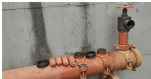
VÁLVULAS ANGULARES RETIRADAS EN CABEZAL
