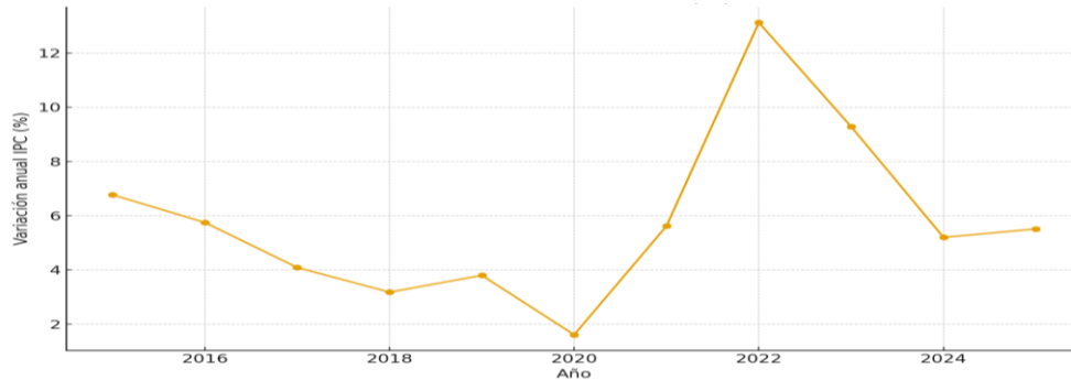
Gráfico 1 Variación anual del IPC 2015 - 2025
