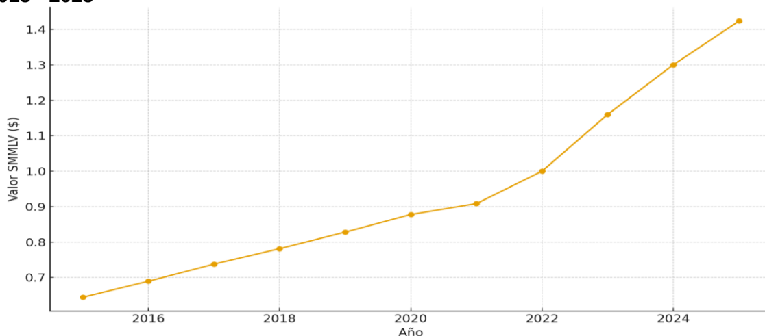
Gráfico 2 Variación Salario Mínimo Mensual Legal Vigente Colombia 2015 - 2025
