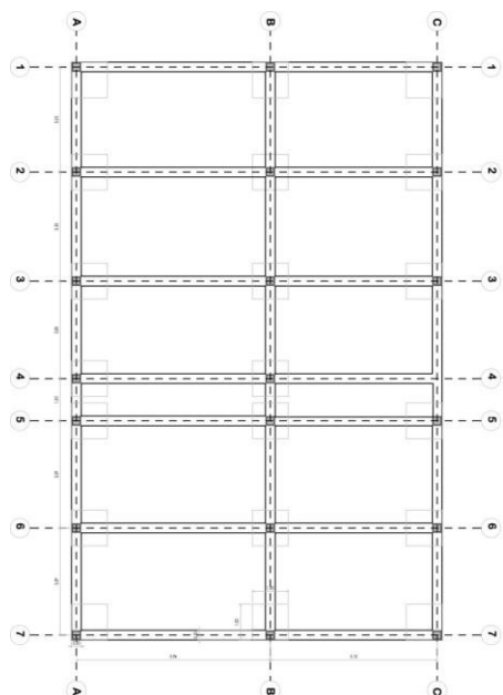
PLANTA DE EJES Y CIMIENTOS DEL GALPON
