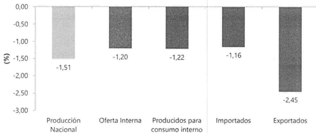
Gráfico 1. Variación mensual de los índices del IPP
