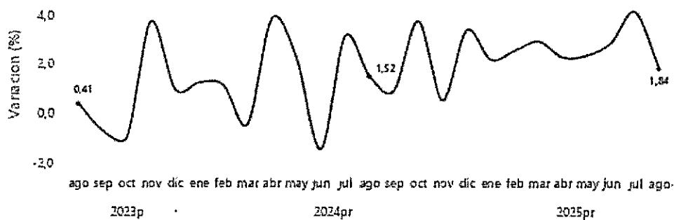
Gráfico 5. Tasa de crecimiento anual del índice del Indicador de Seguimiento a la Economía (ISE) Serie ajustada por efecto estacional y calendario 2023 p - 2025 pr (agosto)
