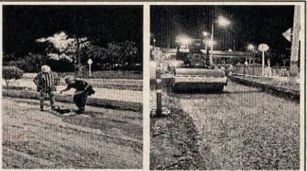
DESCRIPCIÓN: Llenos, compactación y nivelación de base granular Carrera 49 - Estación del Metro.
