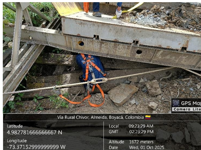
Foto 2: Trabajo de anclaje de la sección del tablero con tirantes para ser izada, se observa personal con elementos de protección personal y de trabajo en alturas.
