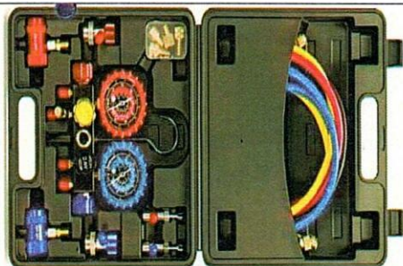
Foto 5: MANÓMETROS
