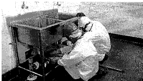
BOSQUEJO DE PUESTA EN FUNCIONAMIENTO DE TRAMPA DE GRASA PORTATIL
