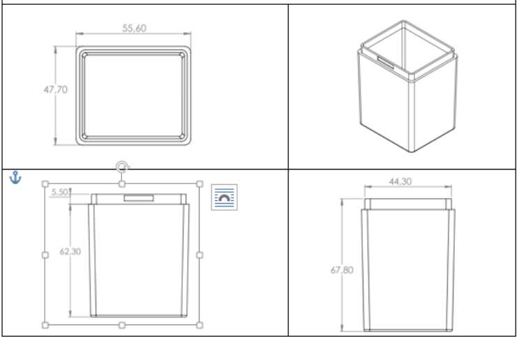
Figura 1. Cajetilla pequeña (mm)
