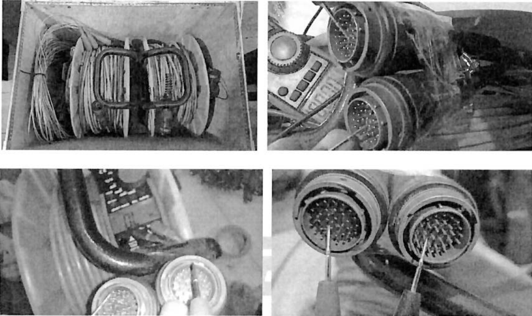
Imagen revisión continuidad pin a pin de los conectores cables de arrastre
