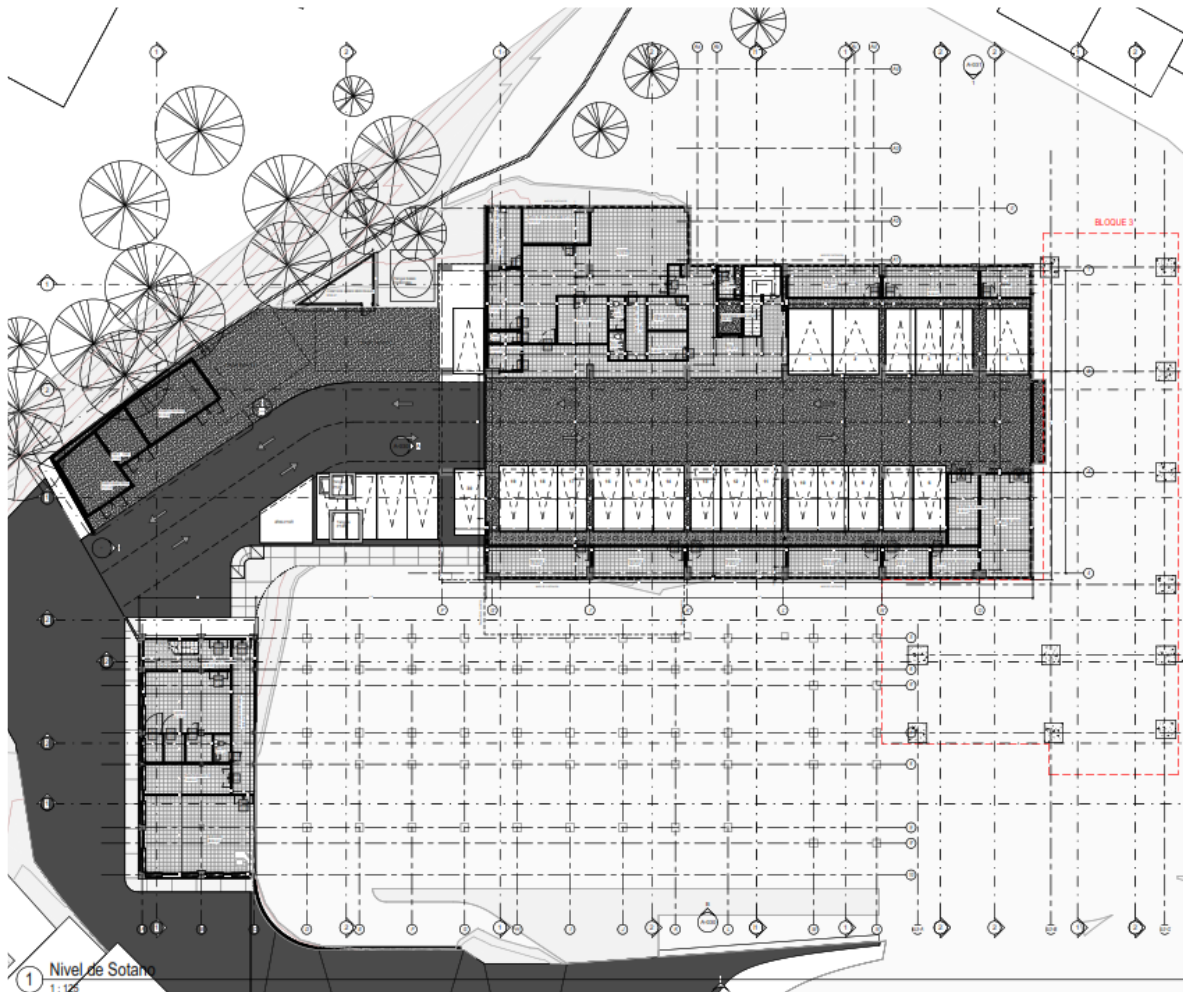
Planta Cubiertas
