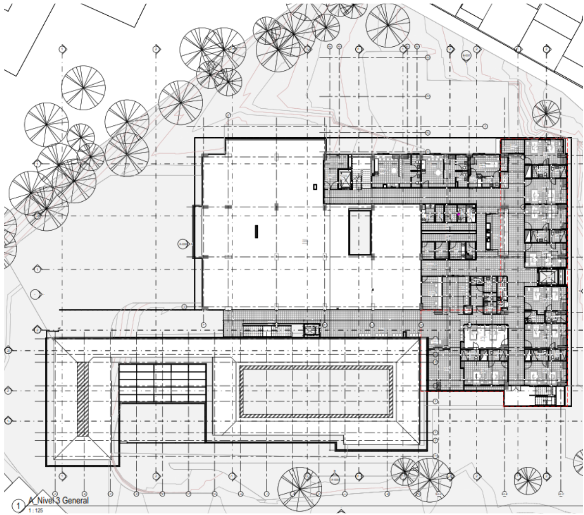
Planta nivel -1
