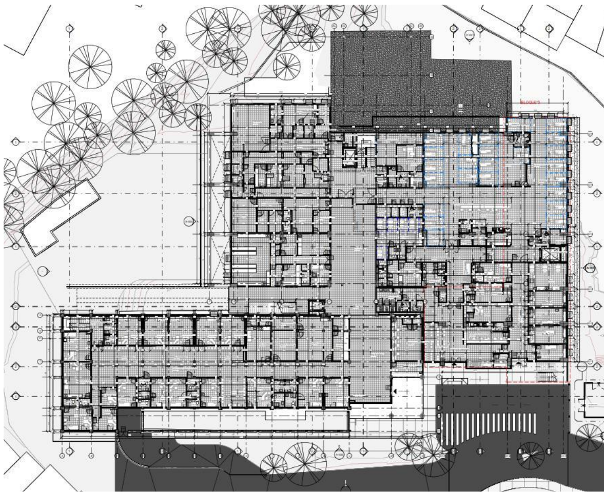
Planta Nivel 2
