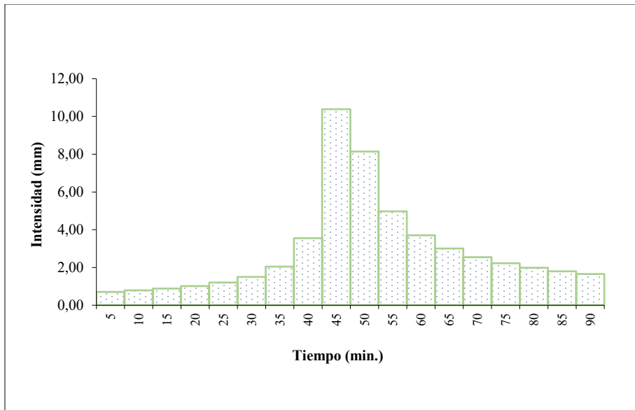
Figura 68. Hietograma de diseño comuna 20TR=15 AÑOS,
