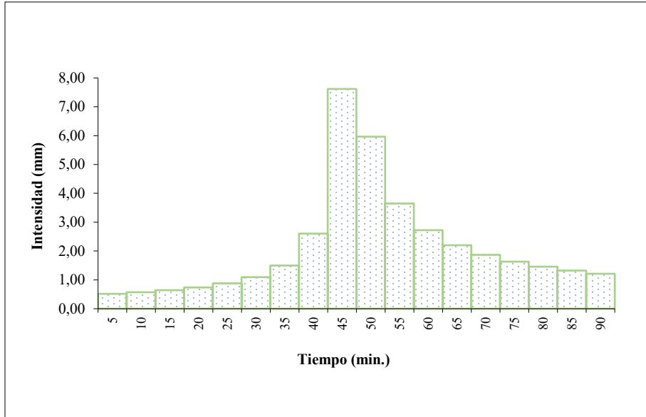
Figura 67. Hietograma de diseño comuna 20 TR=2,33 años
