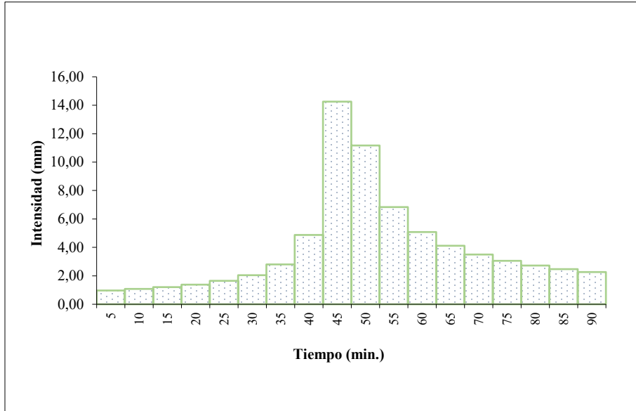
Figura 69. Hietograma de diseño comuna 20 TR=100 AÑOS,
