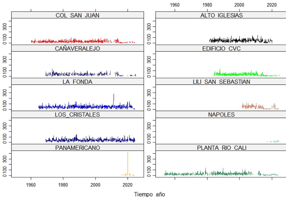
Figura 39, Extensión de los registros de la precipitación máxima diaria en las diferentes estaciones,
