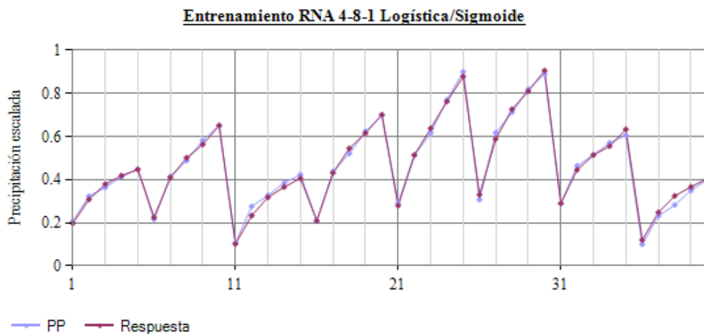
Figura 60, Gráfica Resultados RNA 4-8-1 Entrenamiento – Simulación PMAX24H,
