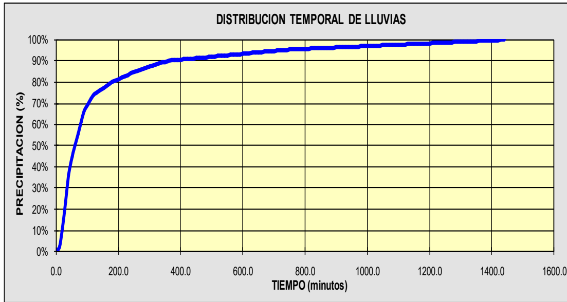
Figura 66, distribución temporal de lluvias promedio para el valle del cauca, Fuente: Infraestructura de servicios públicos fideicomiso Las Vegas, Ciudad Meléndez, Valle de Lili Oriental (HIDRO-OCCIDENTE S.A, 2008),
