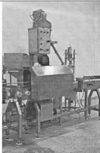
Equipo 3: Túnel de secado con dos turbinas (Superior e inferior)
