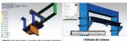
Distribución de carga - montaje de soportes laterales
