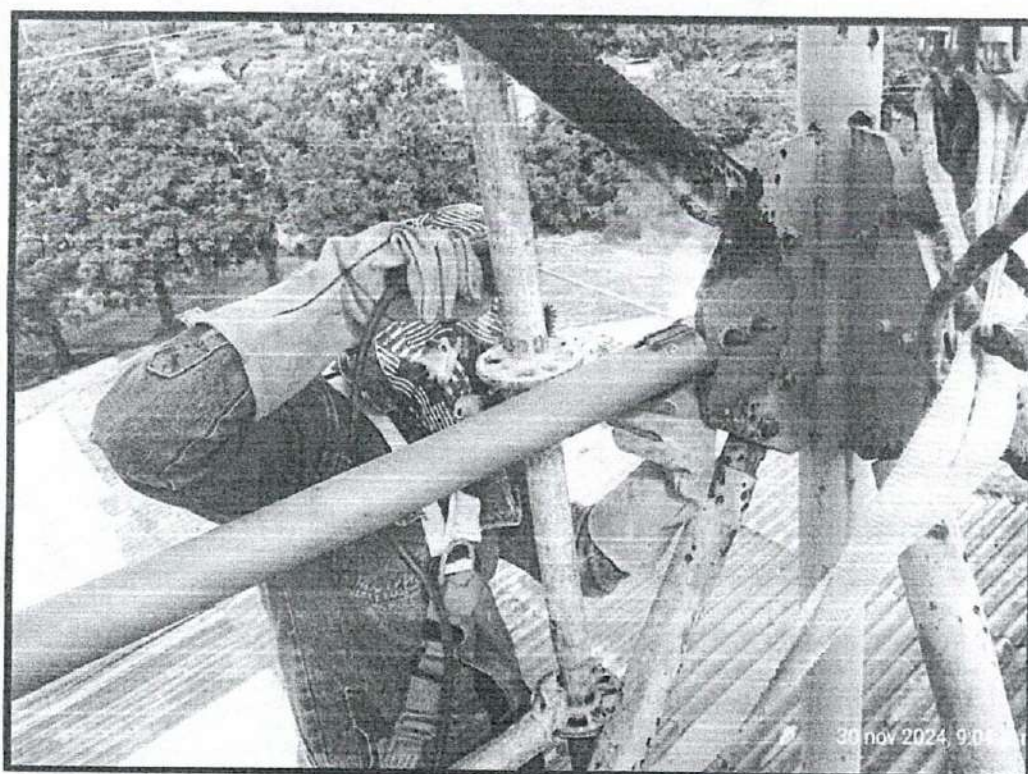
Reforzamiento torre estructural binacional
