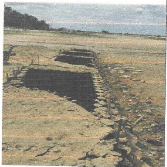
Fotografía 7. Relleno de geocelda 150 mm.
