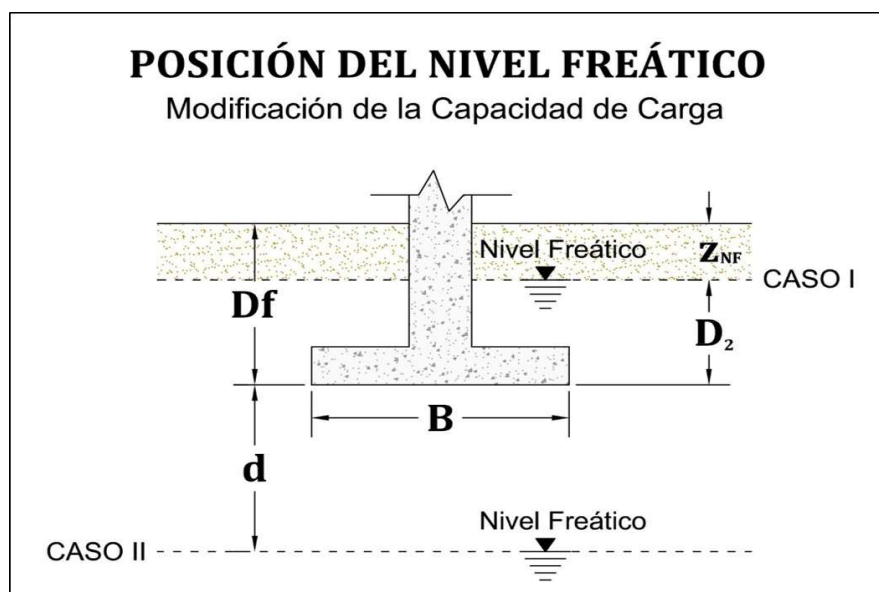
Figura 2.1 - Modificación de la Capacidad de Carga Admisible con el NF.
