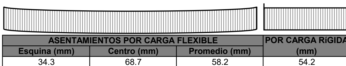
Figura 8.3 - Asentamientos elásticos para la Carga Máxima Admisible de Servicio
