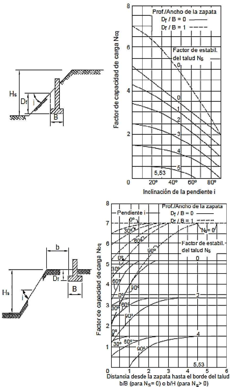
Fig. 6.2 - Factores de capacidad de apoyo para estructuras en o junto a laderas
