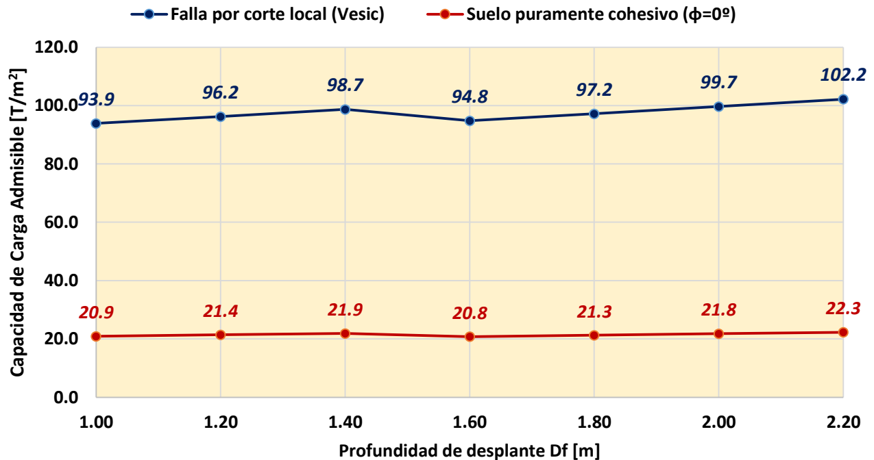
Fig. 7.1 - Estados Límites de Resistencia
