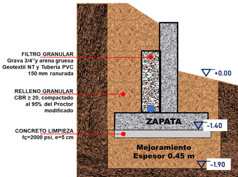
Fig. 12.1 - Esquema de la cimentación
