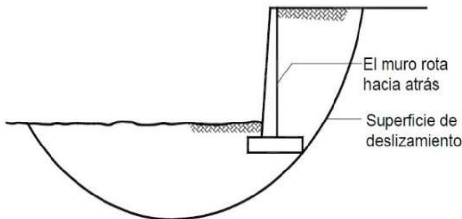
Fig. 6.1 - Falla por Estabilidad Global
