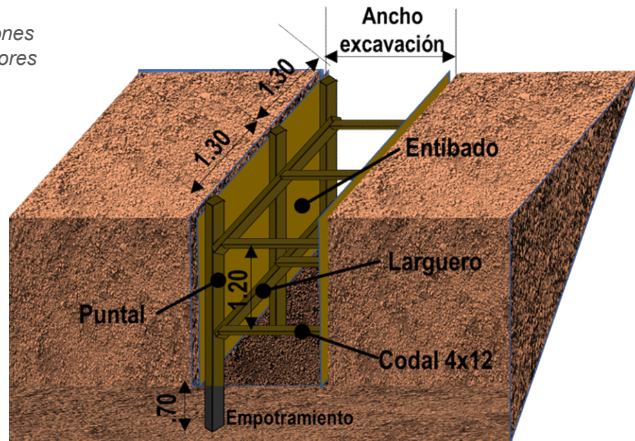
Fig. 12.2 - Recomendaciones de excavación para profundidades mayores a la crítica
