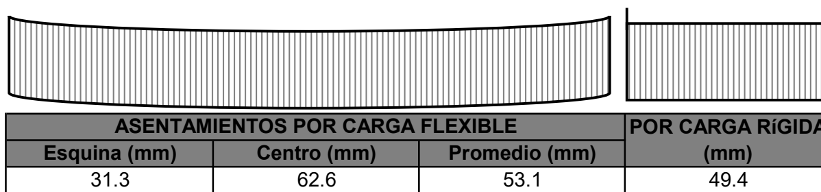
Fig. 8.1 - Asentamientos por carga flexible y rígida
