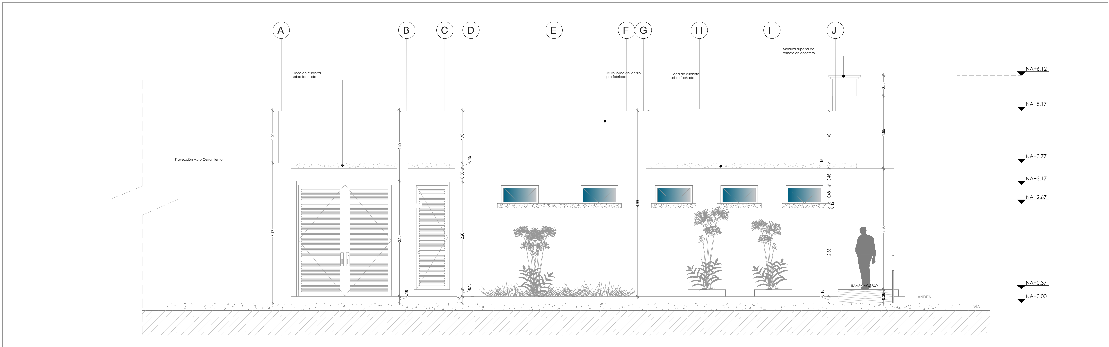
FACHADA LATERAL IZQUIERDA-PROPUESTA
