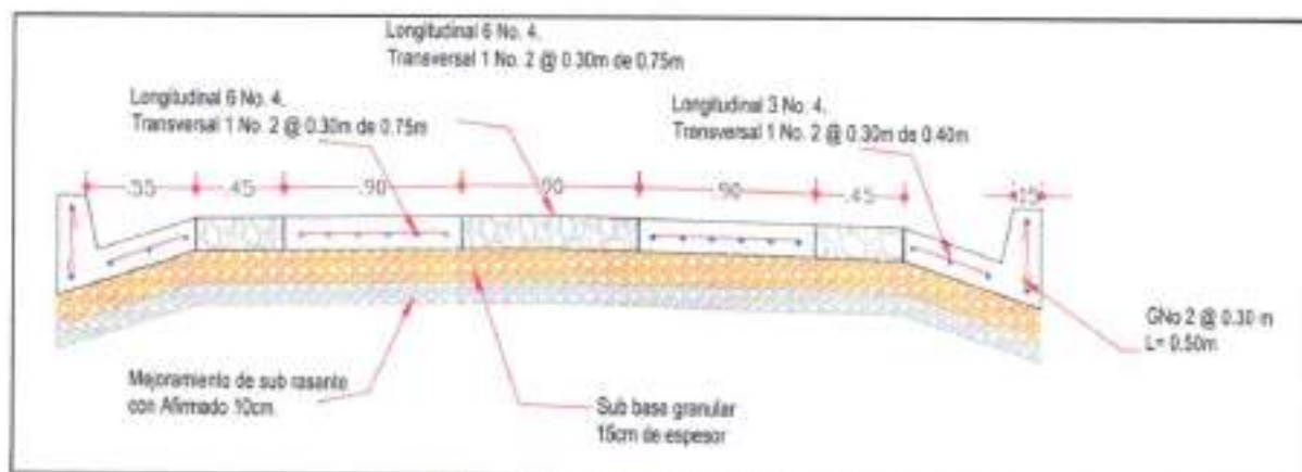
Ilustración 11. Especificación de la vía construida.
