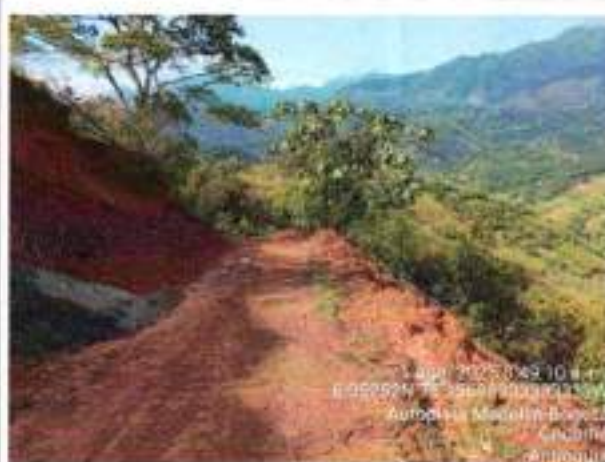
Foto No. 01: Evolución de la rasante a causa de las aguas lluvias. Estado 1, tramo # 3.
