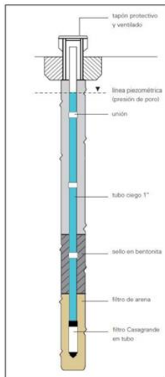
Figura 10. Esquema del piezómetro tipo Casagrande (Fuente: SISGEO, 2016)
