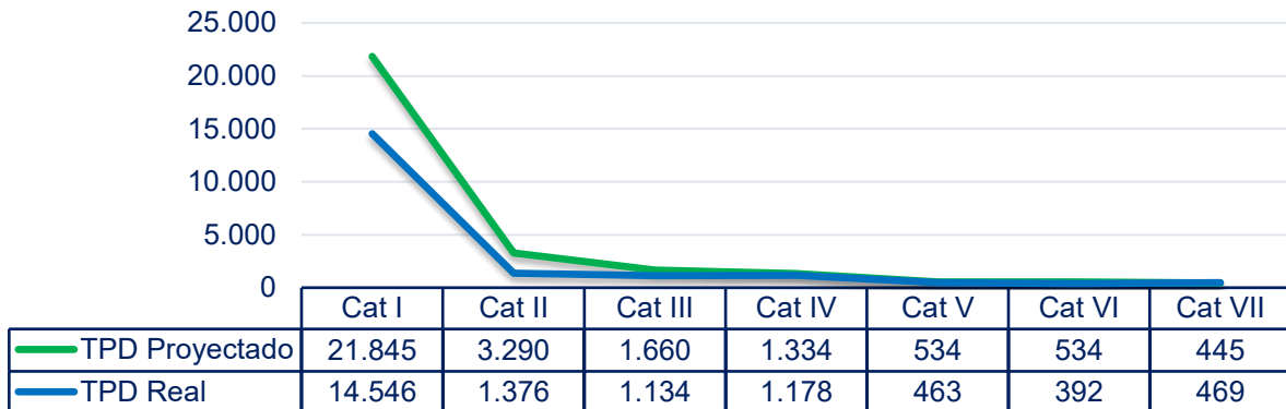
Ilustración 29 TPD por Categoría real y proyectado - Peaje Siberia Fuente: Elaboración propia
