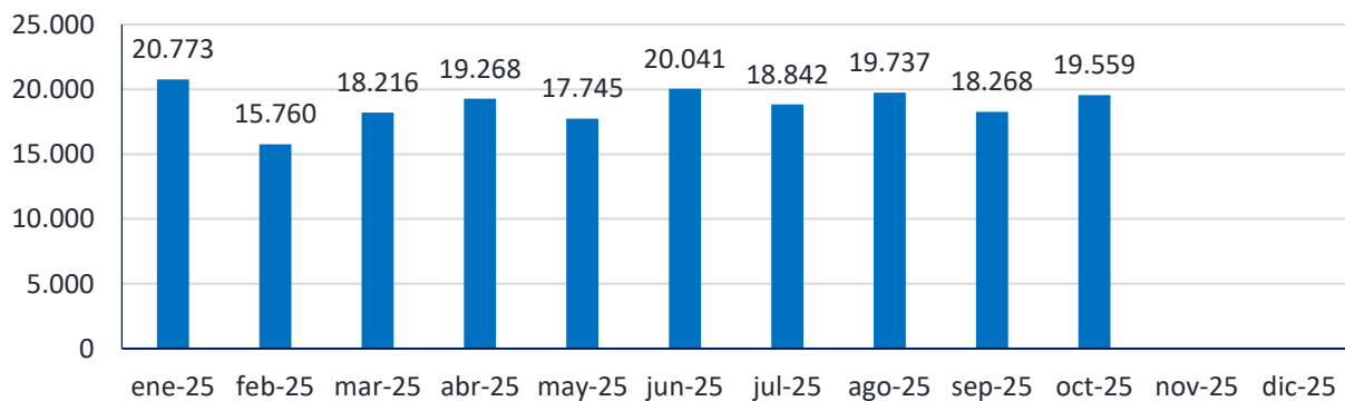
Ilustración 31 TDP por Mes, Año 2025 – Peaje Siberia Fuente: Elaboración propia
