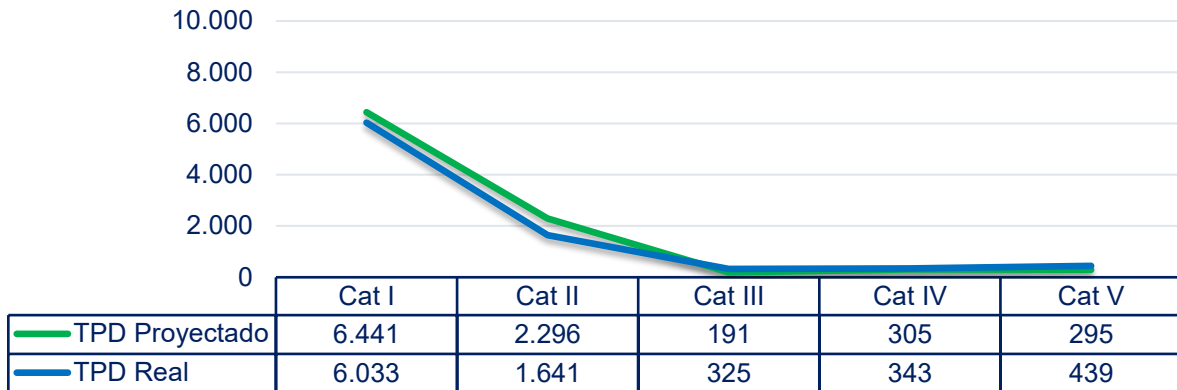
Ilustración 34 TDP por Categoría real y proyectado - Peaje Caiquero Fuente: Elaboración propia
