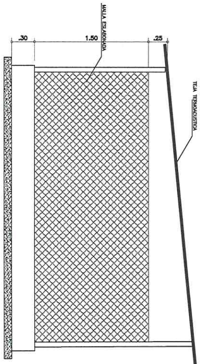
VISTA LATERAL CERRAMIENTO TIPO EN MALLA ESLABONADA
