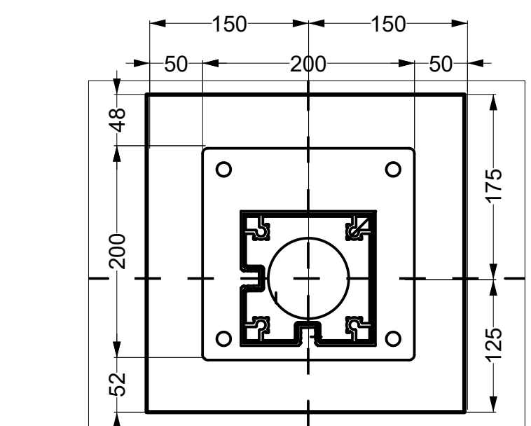
PLACA BASE EJE 7C
