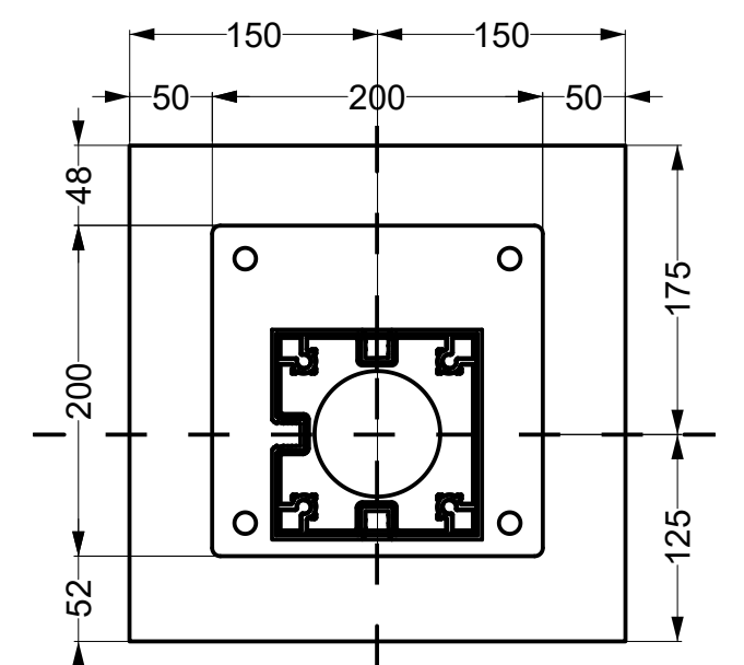
PLACA BASE EJE 3C
