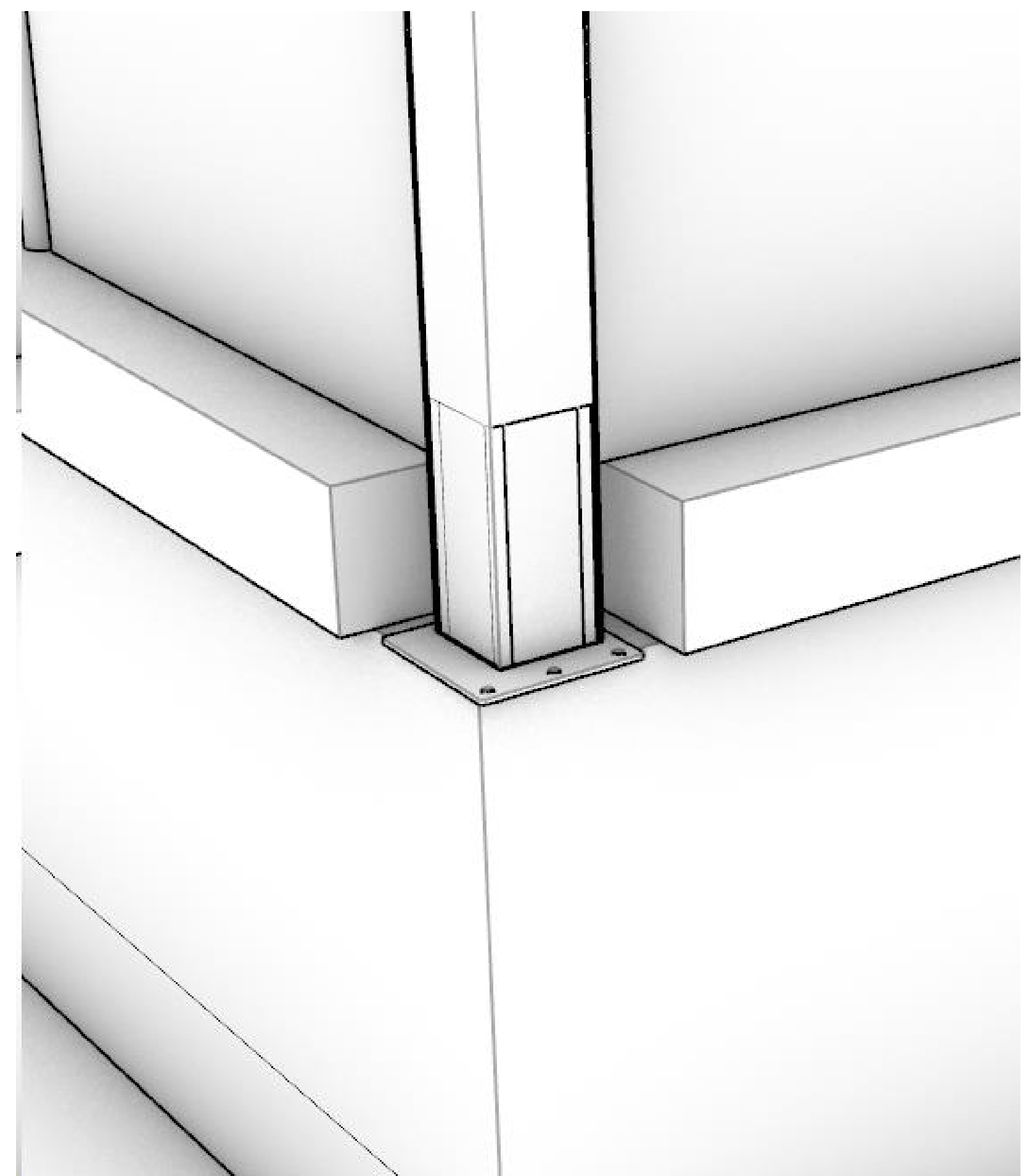
DETALLE CORTE REQUERIDO EN ALFAJIA (DEBE SER REALIZADO POR CLIENTE)
