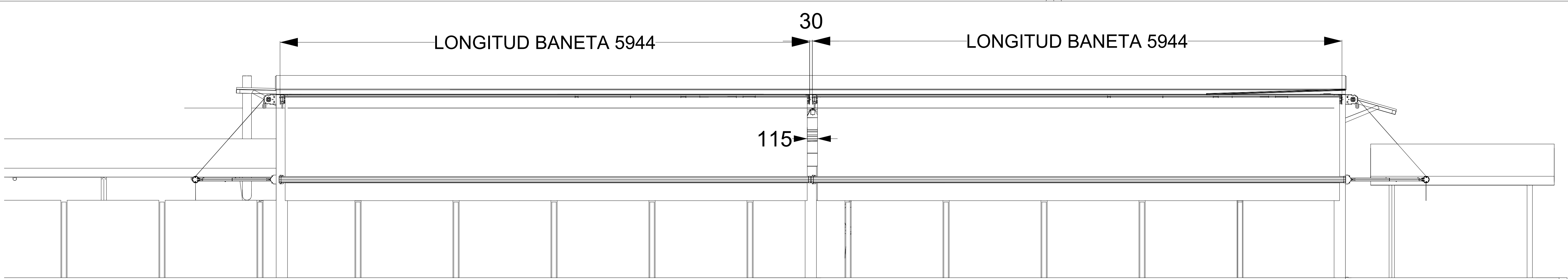
VISTA FRONTAL BANETAS 1 Y 2
