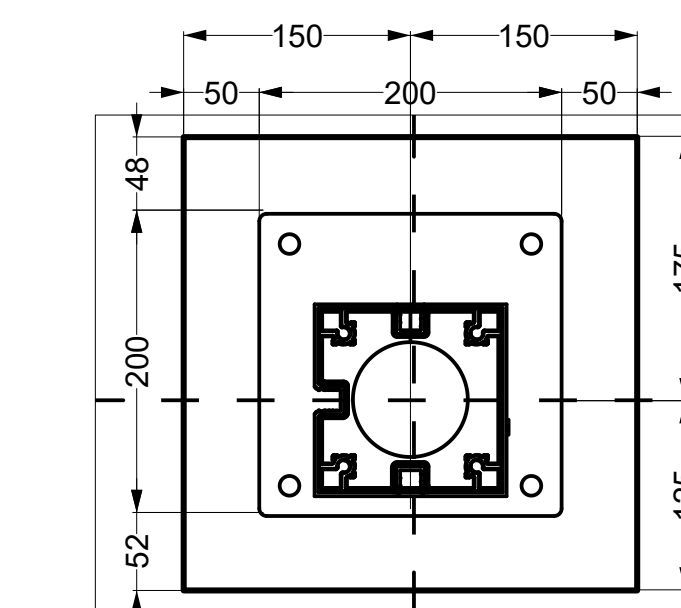
PLACA BASE EJE 6C
