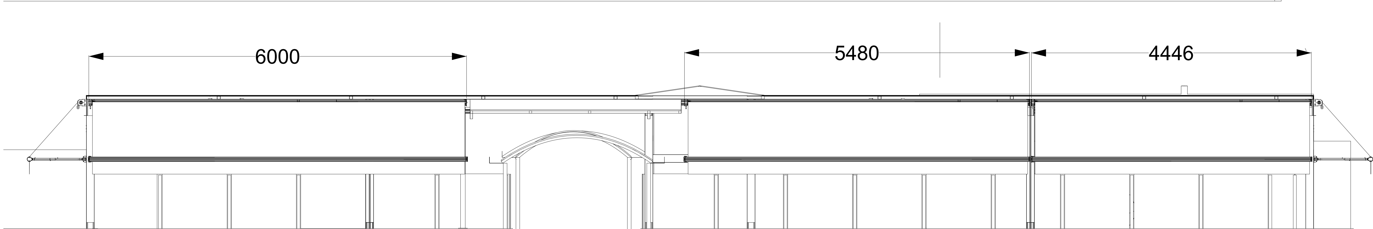
VISTA FRONTAL BANETAS 1 Y 2
