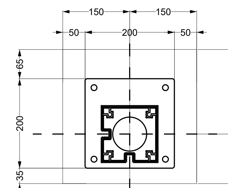
PLACA BASE EJE 7A
