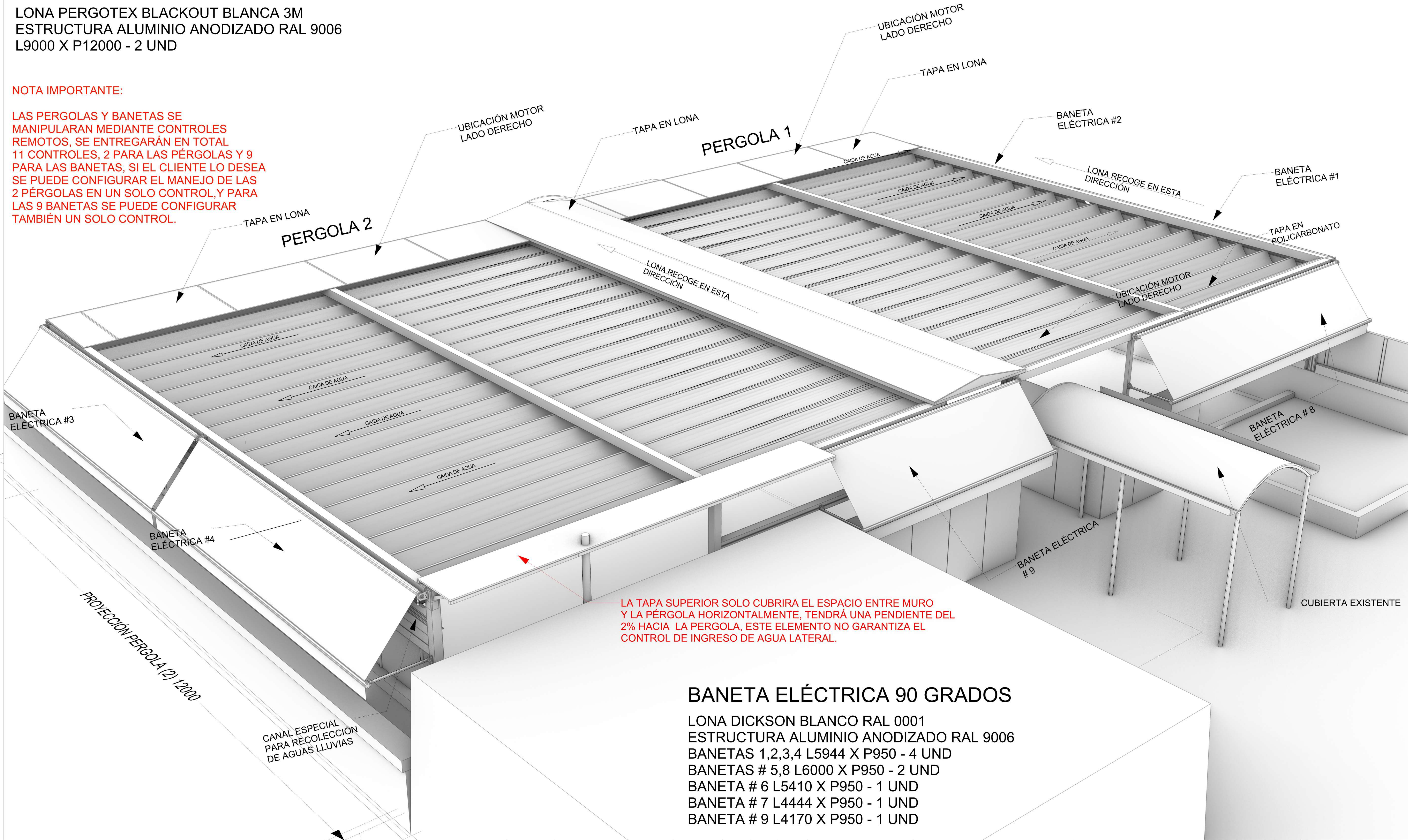
VISTA GENERAL COSTADO OCCIDENTE
