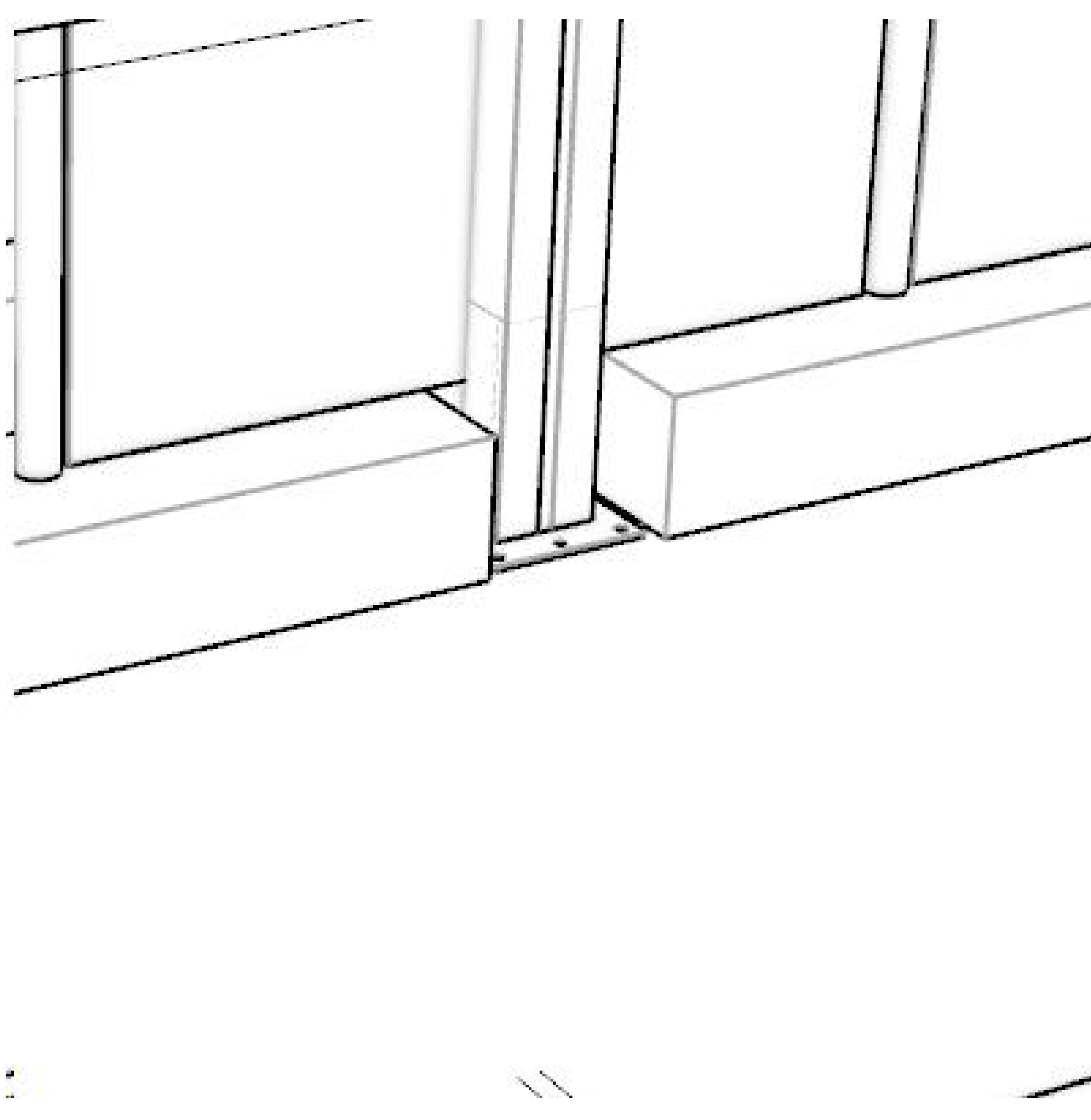
DETALLE CORTE REQUERIDO EN ALFAJIA (DEBE SER REALIZADO POR CLIENTE)
