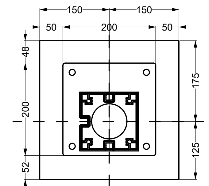
PLACA BASE EJE 2C
