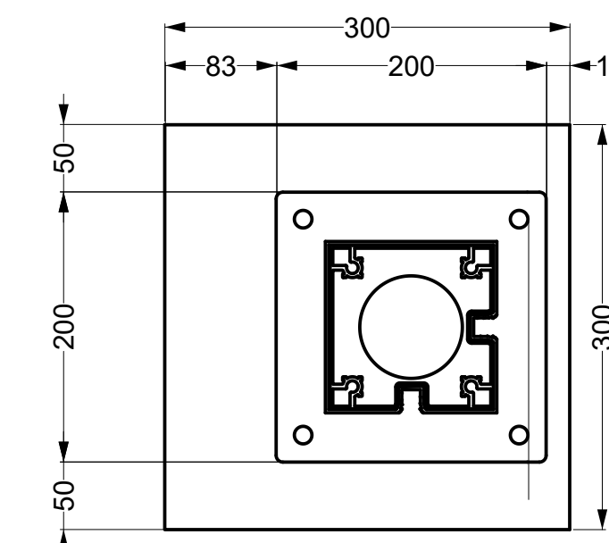
PLACA BASE EJE 1C
