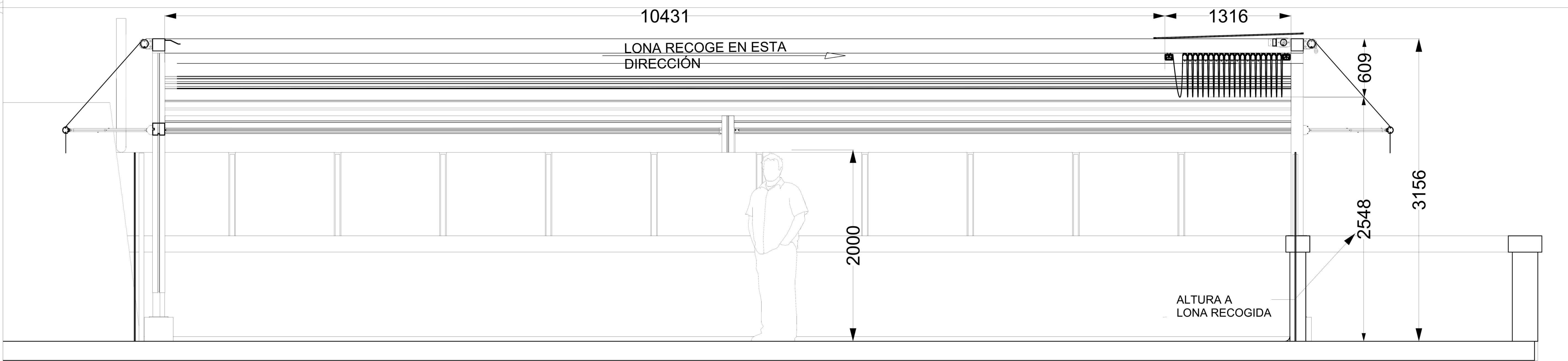
VISTA LATERAL LONA RECOGIDA
