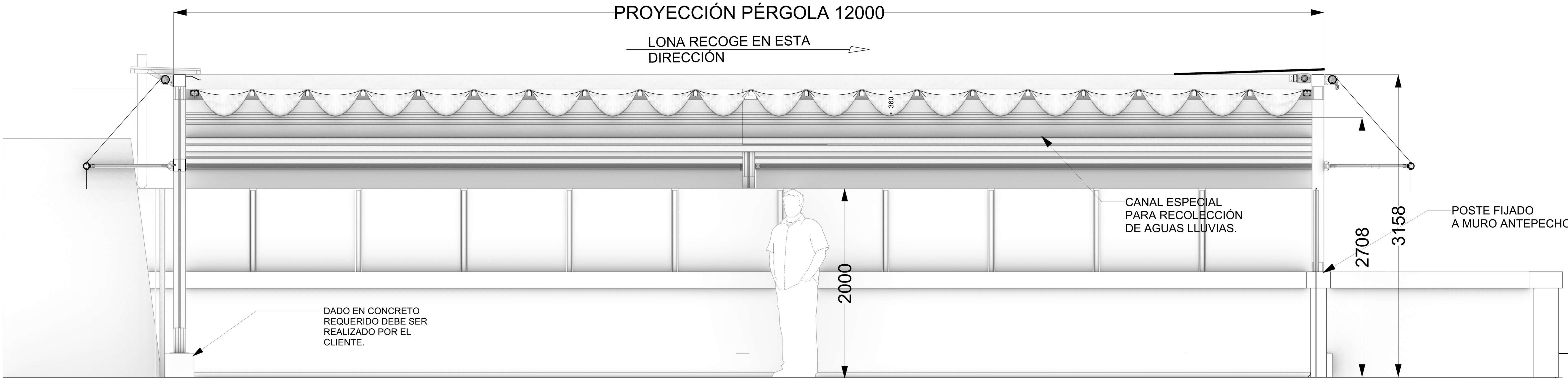
VISTA LATERAL LONA EXTENDIDA
