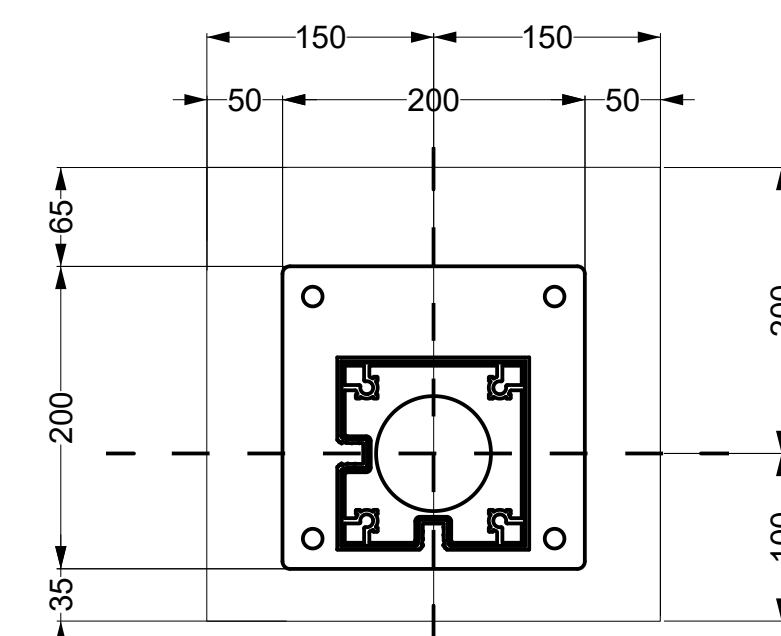
PLACA BASE EJE 7B
