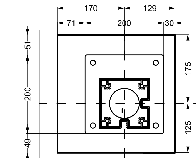
PLACA BASE EJE 4C
